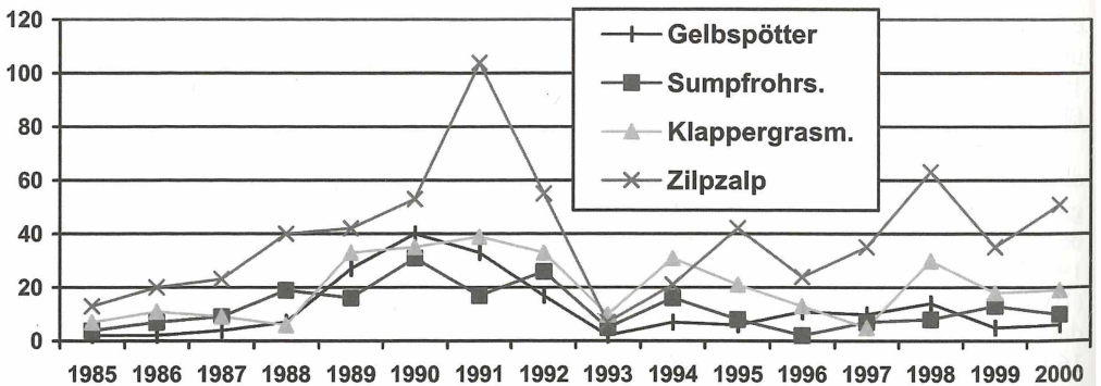
Abb. 3. Bei den hier vorgestellten Arten fiel auf, daß diese kurz nach Sukzessionsbeginn Bestandsmaxima erreichten, also wahrscheinlich dieses bestimmte Stadium bevorzugten.
