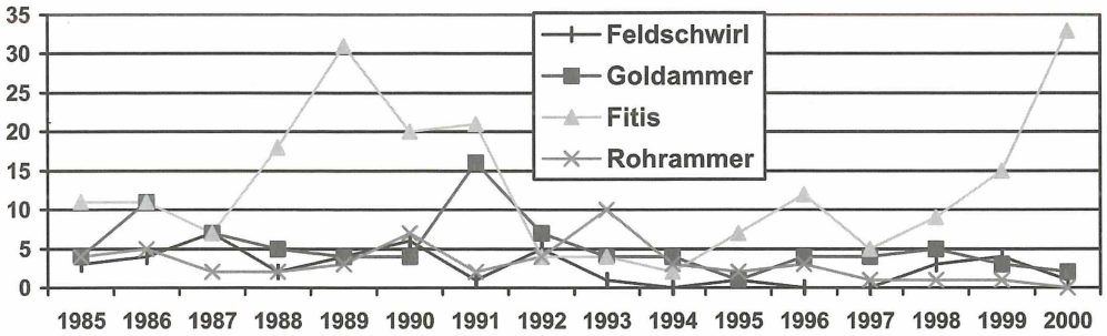
Abb. 4. Alle vier Arten wiesen über die gesamten 16 Untersuchungsjahre keinen deutlichen Bestandstrend auf, für den auch keine Signifikanz nachgewiesen werden konnte. Gleiches gilt für die nicht dargestellten Arten Heckenbraunelle, Neuntöter und Singdrossel.
