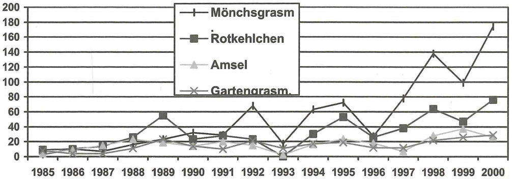
Abb. 2. Die hier dargestellte Entwicklung der Fangzahlen zeigt bei allen vier Arten einen signifikanten Trend: Mönchsgrasmücke Regressionskoeffizient 8,84, Korrelationskoeffizient 0,85, Rotkehlchen 3,05/0,68, Amsel 1,03/0,53 und Gartengrasmücke 0,99/0,63. Bei Mönchsgrasmücke und Rotkehlchen ist in den letzten Untersuchungsjahren besonders die Anzahl der Durchzügler gestiegen. Ebenfalls nicht zufällig sind die hier nicht dargestellten Trends von Gimpel (0,89/0,76) und Nachtigall (0,69/0,83).
