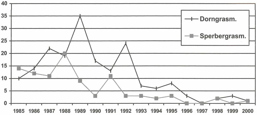
Abb. 1. Dorn- und Sperbergrasmücke zeigen einen deutlichen negativen Bestandstrend (Regressionskoeffizient -1,45 bzw. -1,06 ). Für die Korrelationskoeffizienten ( -0,71 bzw. -0,78 ) konnte mittels t-Test bei einer Irrtumswahrscheinlichkeit von 5% (gleicher Test für die Trends in Abbildung 2 und 4 verwendet) Signifikanz nachgewiesen werden.
