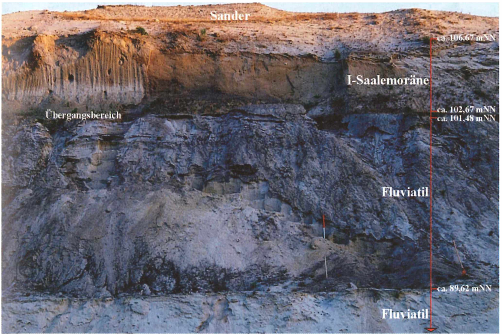
Bild 1. Übersicht über das Profil Greifenhain A.
