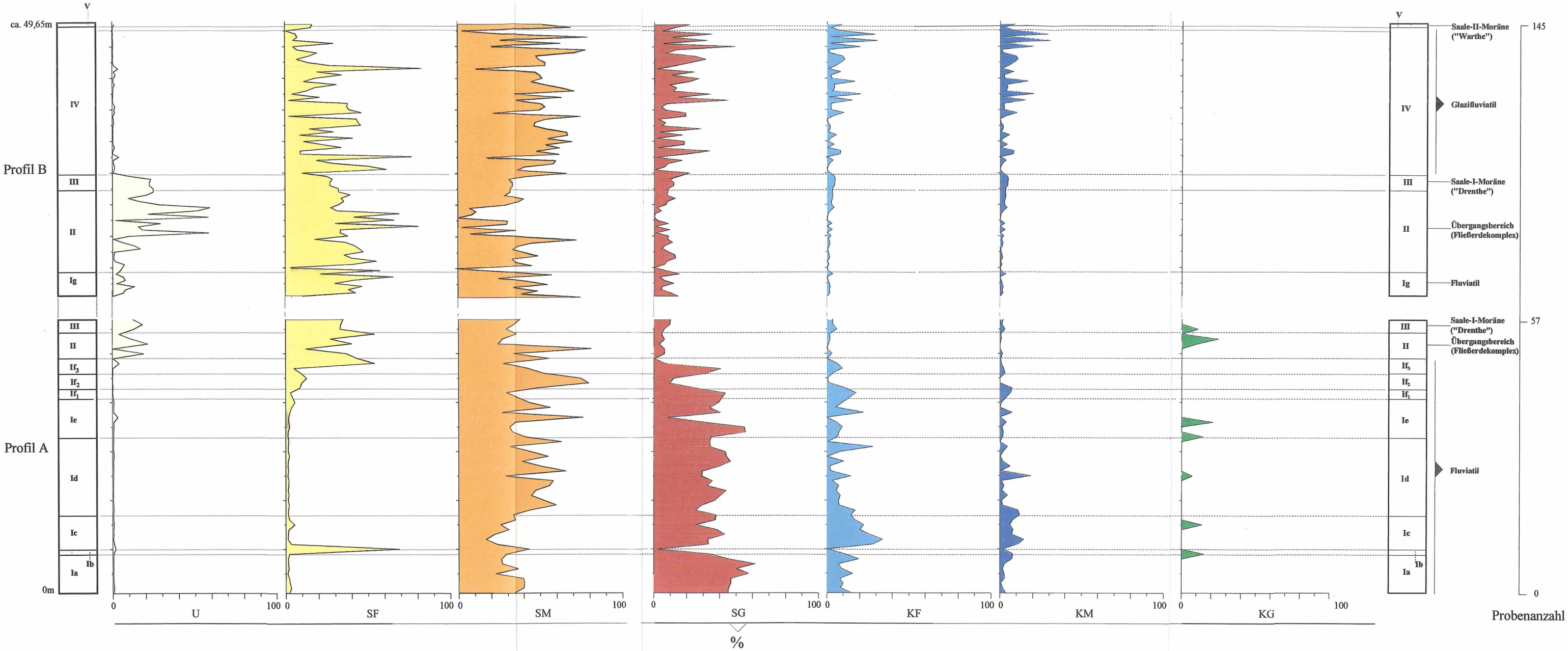
Abb. 9. Korngrößenfraktionen des Saalekomplexes im Tagebau Greifenhain
