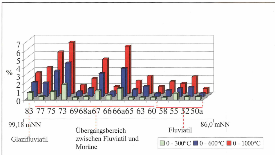
Abb. 8. Glühverlust des Profils Greifenhain B.
