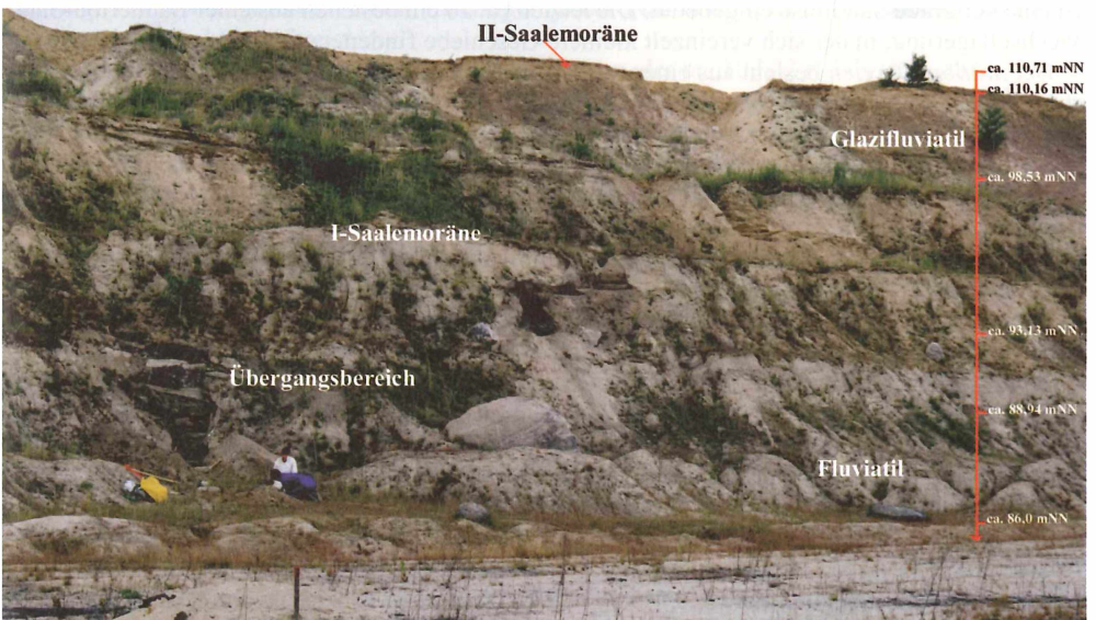
Bild 3. Übersicht über das Profil Greifenhain B.
