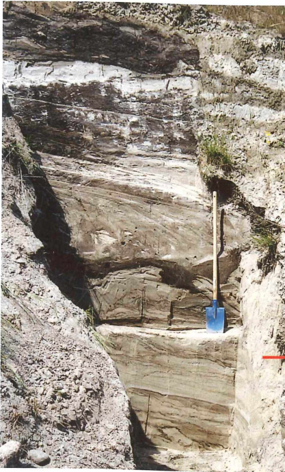
Bild 4. Überblick über den Abschnitt II.
