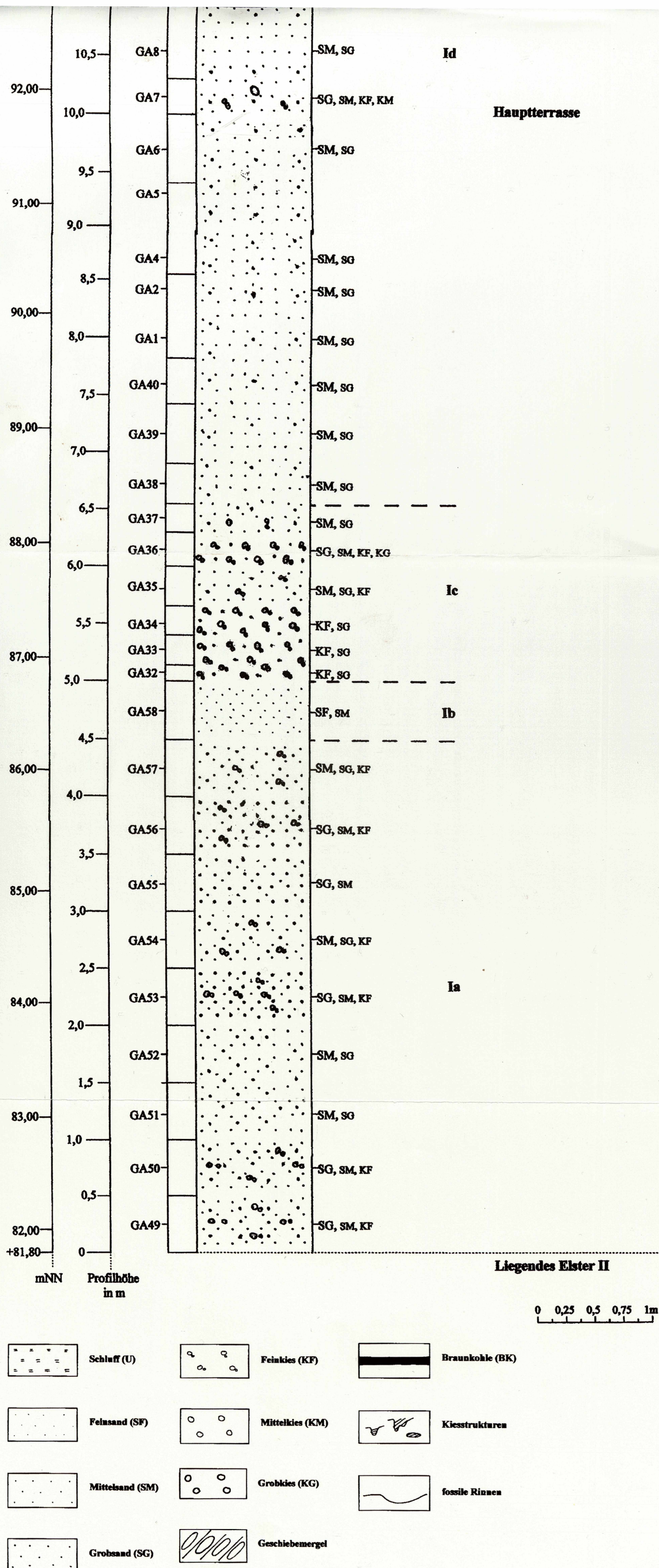
Abb. 3. Profilschnitt Greifenhain A (Fluviatil)
