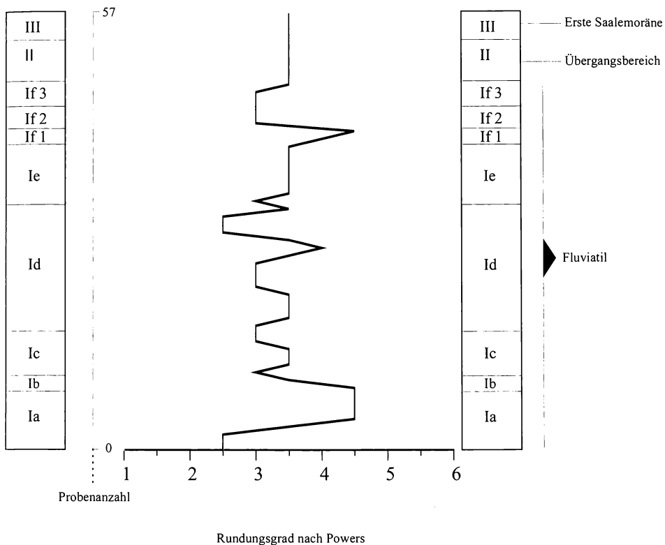
Abb. 4. Darstellung des Rundungsgrades nach Powers im Profil Greifenhain A.
