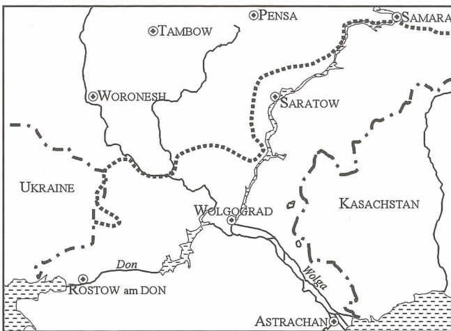
Abb. 1. Südliche Grenze des Verbreitungsareals der Waldsteppenotter ( Vipera nikolskii ) im europäischen Teil Rußlands
