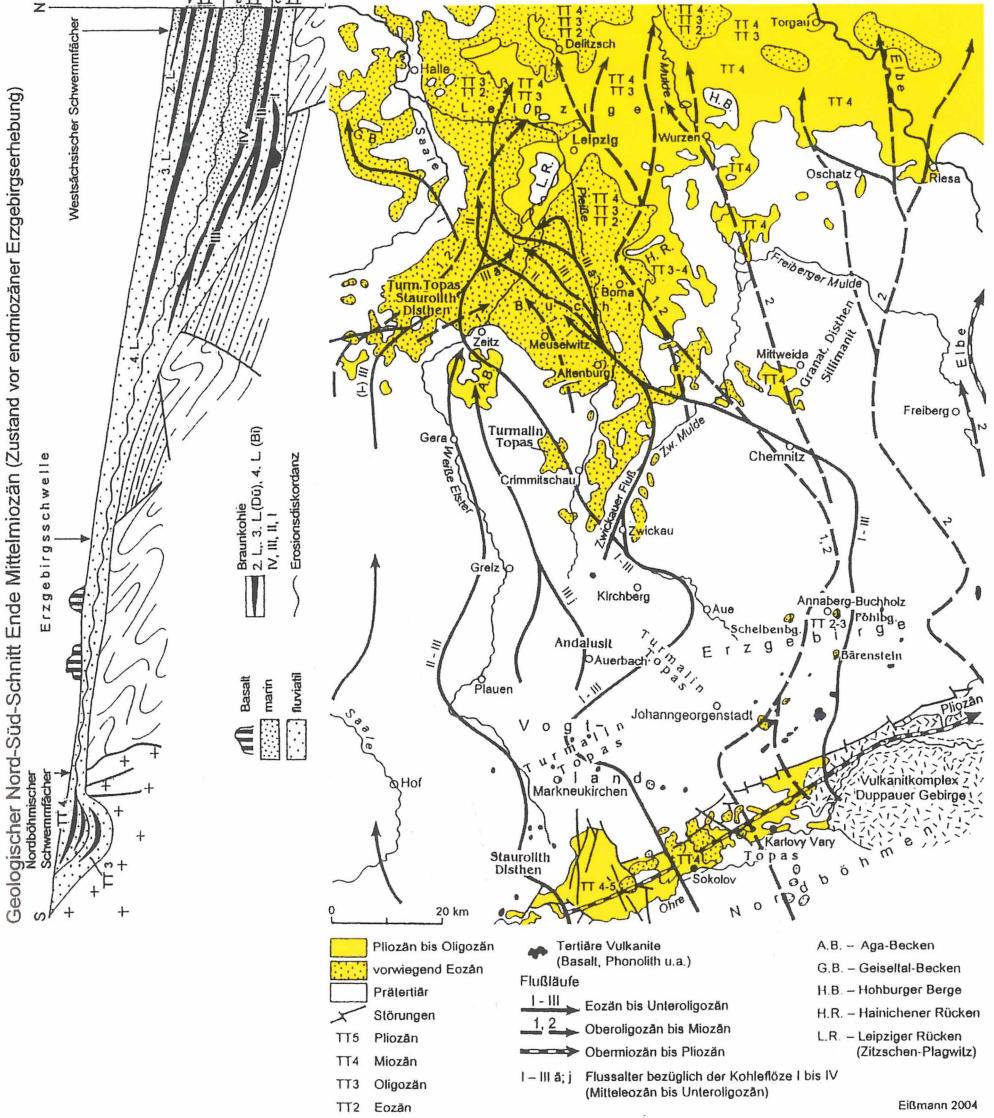
Abb. 4. Nordböhmisches und westsächsisches binnenländisches bis deltaoides (Abb. 5) und ästuaries (zeitengeprägtes) Flußsystem im älteren (Oligozän, Eozän) und jüngeren (Miozän) Tertiär. Mit dem Aufstieg des Erzgebirges im höheren Miozän werden die Abflüsse über das heutige Gebirge blockiert und große Teile Westböhmens über die heutige Elberegion entwässert. Das moderne, heutige Einzugsgebiet entsteht. (Eißmann 1968, 1975 ergänzt)
