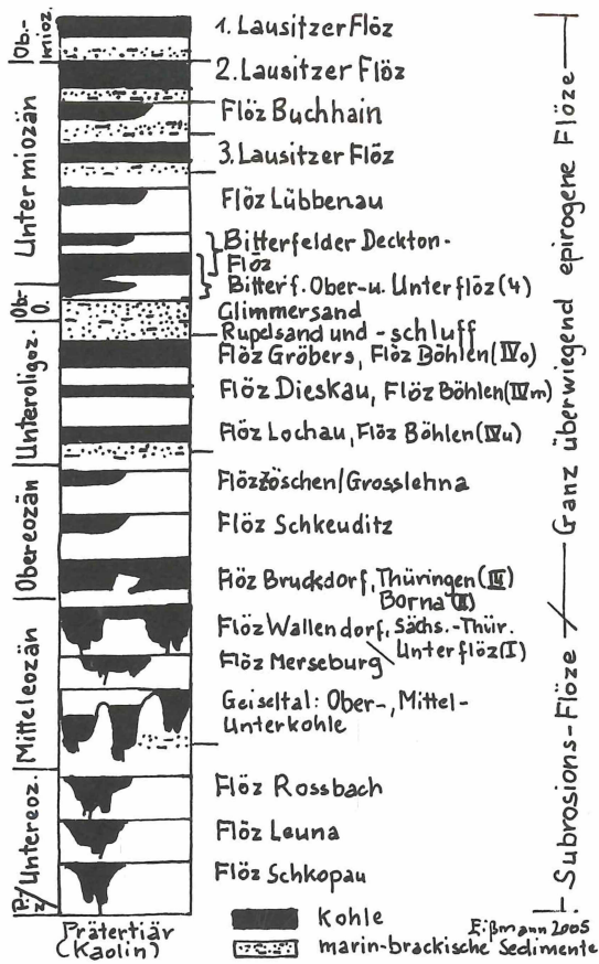
Abb. 3. Braunkohlenflöze und Meeresablagerungen im Tertiär vom Harzvorland bis zur Oder und Neiße.
