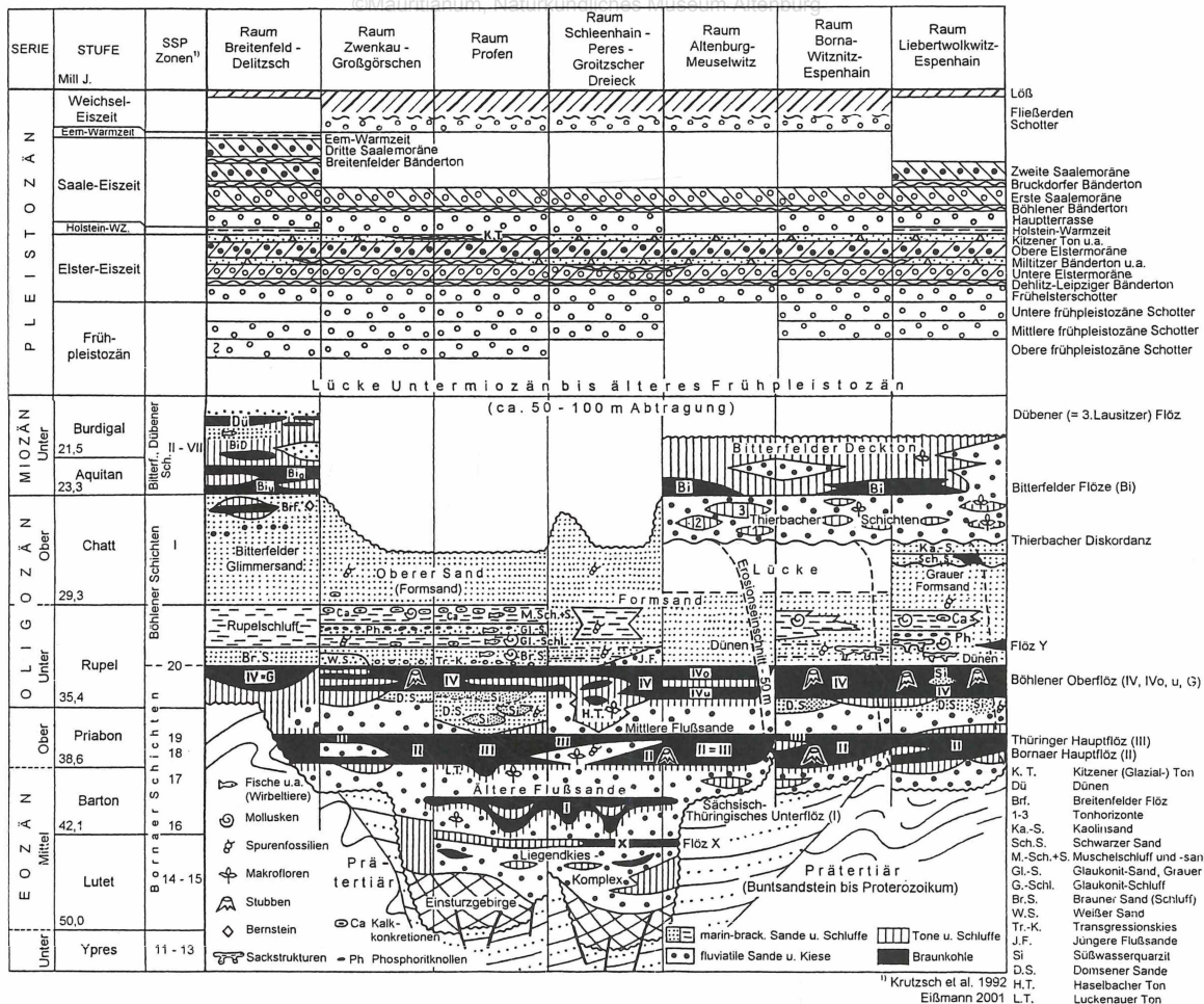
Abb. 1. Quartär (stark vereinfacht) und Tertiär wichtiger durch Braunkohlentagebaue erschlossener Sektionen der mittleren und südlichen („Weißelsterbecken“) Leipziger Tieflandsbucht.
