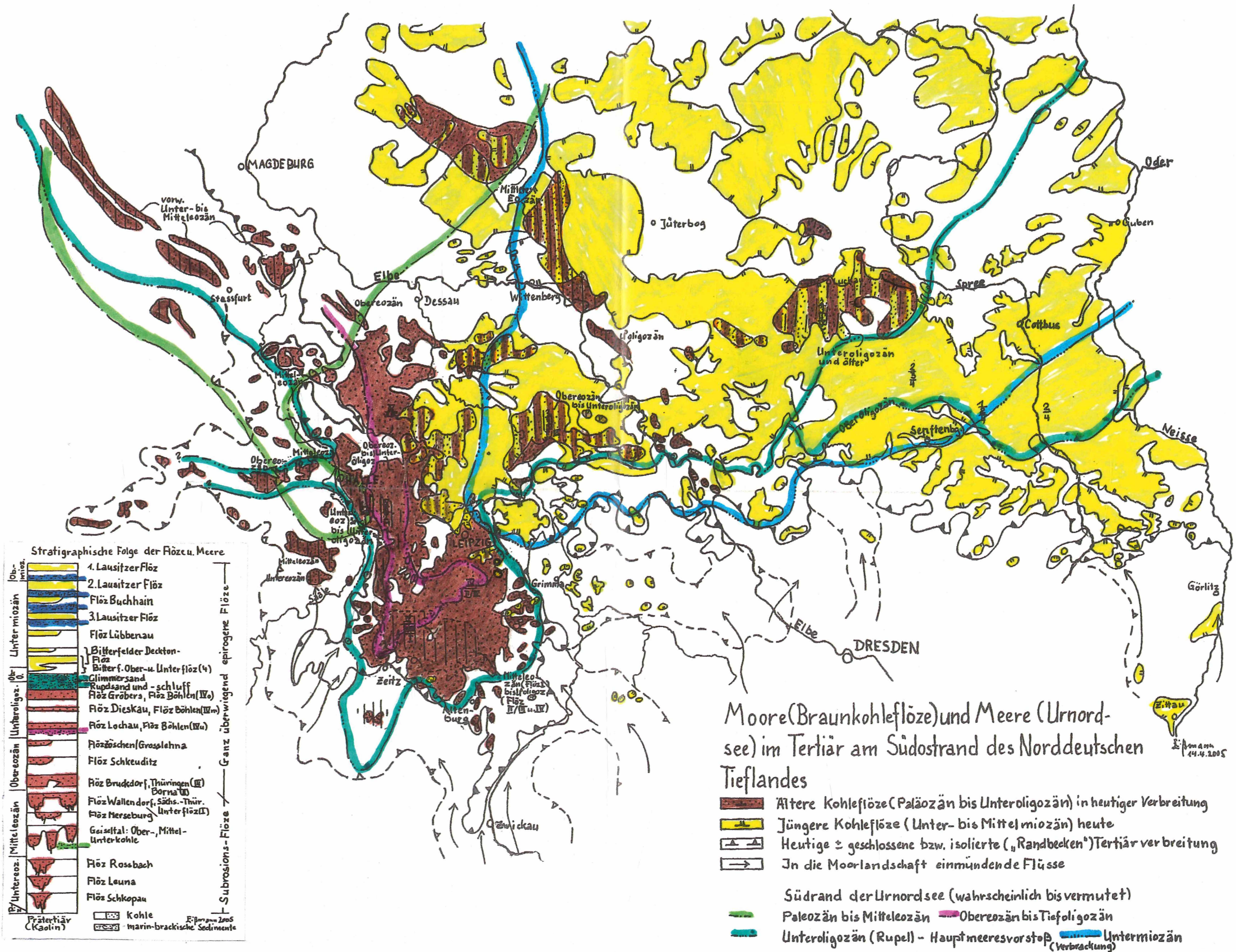
Abb. 6. zu L. EISSMANN: Graphische Kompilationen zum Tertiär Mitteldeutschlands (Paralipomena I). – Mauritianum (Altenburg) 19 (2005) 2, S. 283–288
