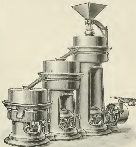
3. Kakaomühle.
