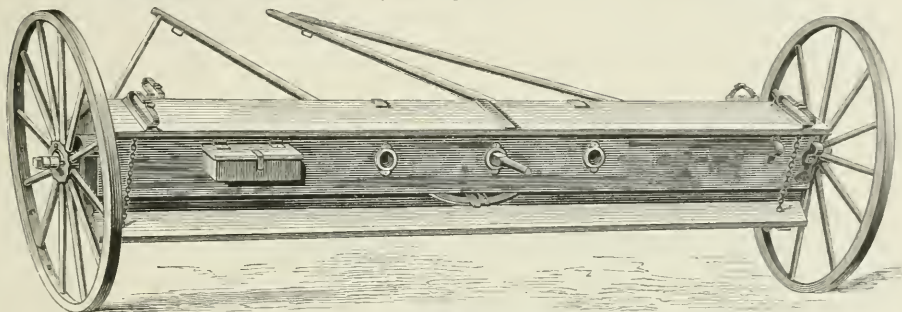
3. Breitsämaschine.
