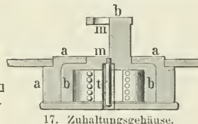
17. Zuhaltungsgehäuse.
