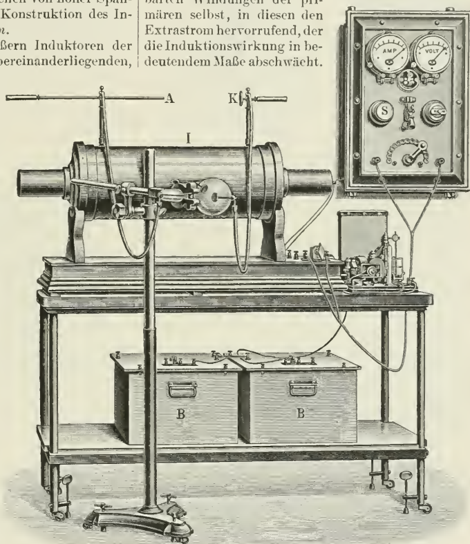
1. Röntgeneinrichtung mit Akkumulatorenbetrieb.
