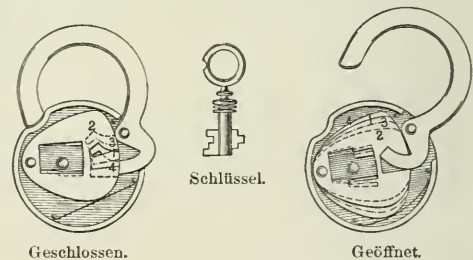
21. Steinkes Vorhängeschloß.
