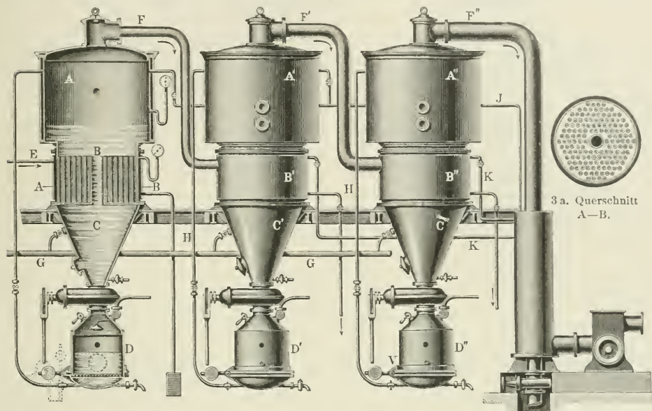
3. Pickseher Verdampfapparat, der erste Körper im Durchschnitt.
