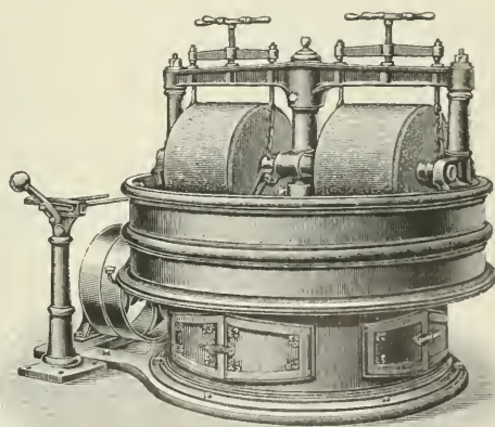
4. Melangeur.
