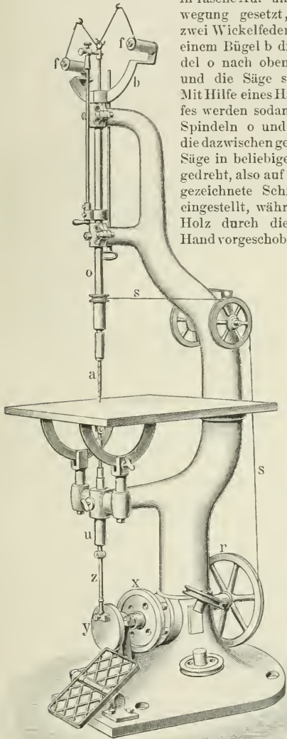
4. Rotativsäge.
