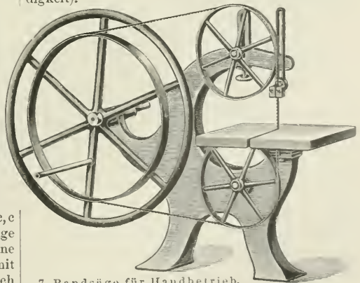
7. Bandsäge für Handbetrieb.
