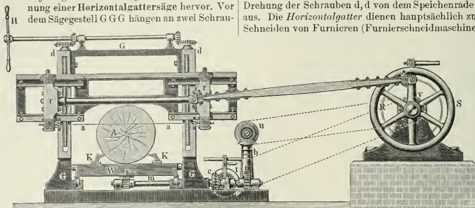
2. Horizontalgattersäge.
