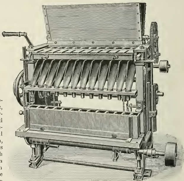
7. Paketfüllmaschine von Wagner.
