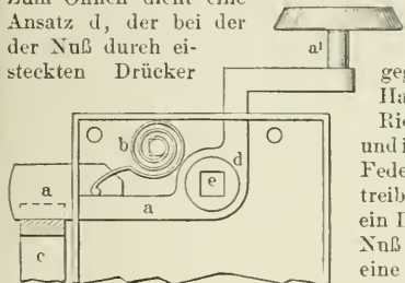
1. Hebende Falle.
