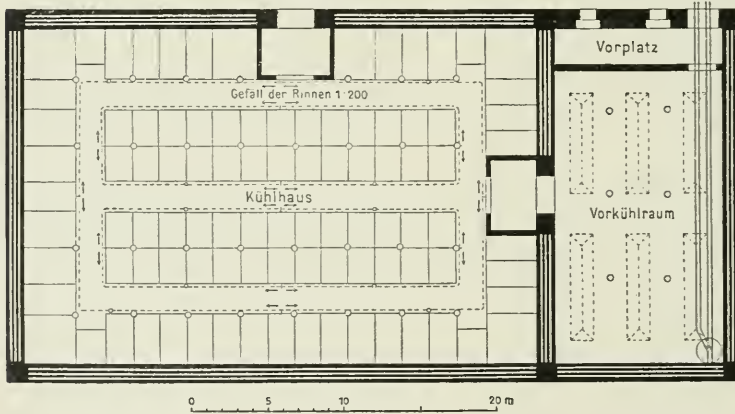
15. Kühlhaus. Grundriß.
