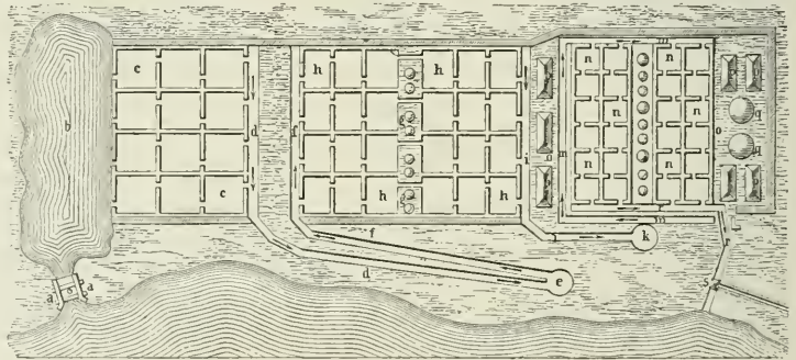
7. Meersaline (Salzgarten).
