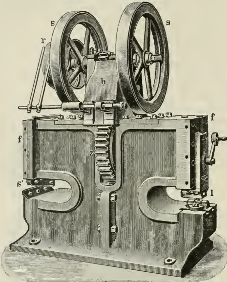
Fig. 4. Vereinigte Loch- und Schermaschine.
