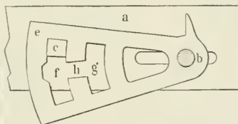
5. Schloßriegel und eine Zuhaltung.
