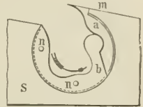
Fig. 9. Auswechselbarer Sägezahn.
