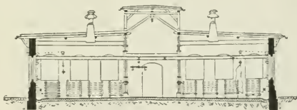
5. Querschnitt C—D.
