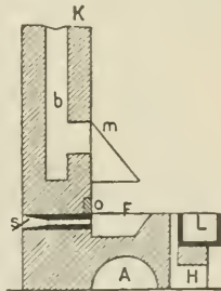
Fig. 1. Schmiedeherb.
