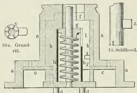
9. Schließzylinder und Zuhaltungen. 8—11. Bramah-Schloß.
