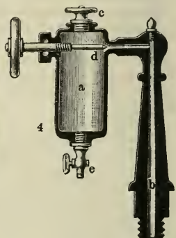
Fig. 3. Schmierhahn. Fig. 4. Kontinuierlich wirkender Schmierapparat.
