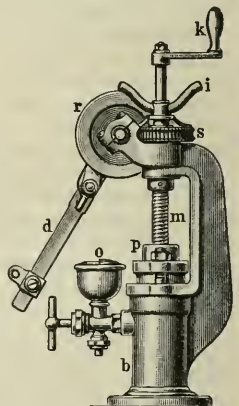
Fig. 5. Schmierpresse.
