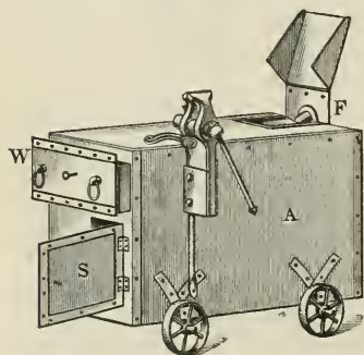
Fig. 3. Feldschmiede.
