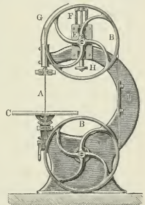
6. Bandsäge.
