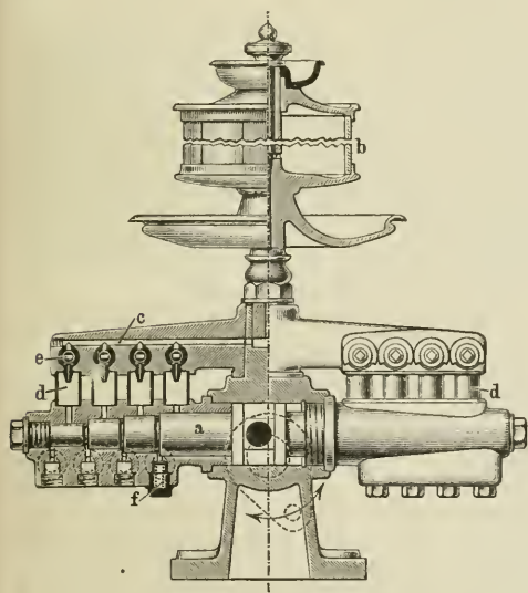
Fig. 6. Schmierpumpe von Lenz.
