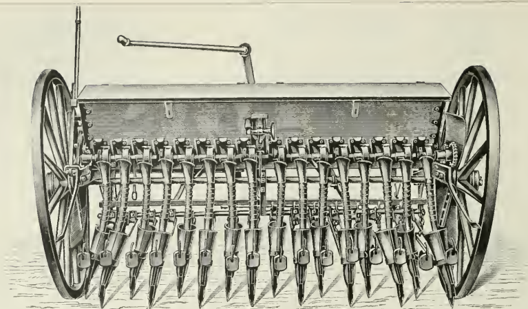
1. Bergdrillmaschine 'Hallensis' von Zimmermann u. Komp., Halle a. S.
