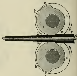
Fig. 4. Pilgerschrittwalzen.
