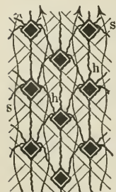
Fig. 2. Einrichtung eines Lattenkamin-Kühlers.
