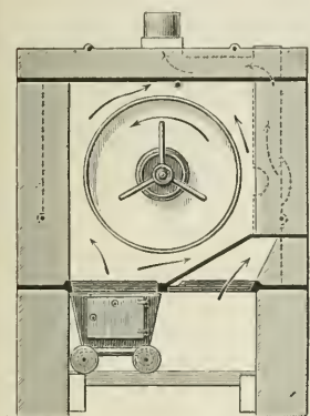
1. Rösttrommel.
