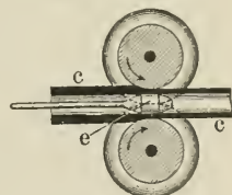
Fig. 2. Rohrwalzwerk.
