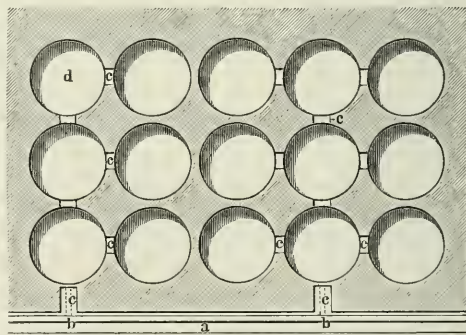
7. Anordnung der Aussolungskessel beim Spritz- verfahren in Schönebeck. a Hauptstrecke, b Süßwasser- leitung, c Querschläge, d Aussolungskessel.
