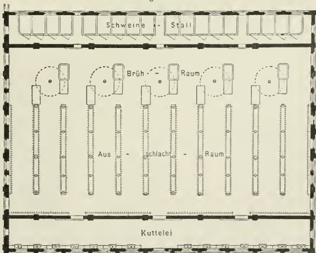
11—13. Schlachthalle für Schweine.
