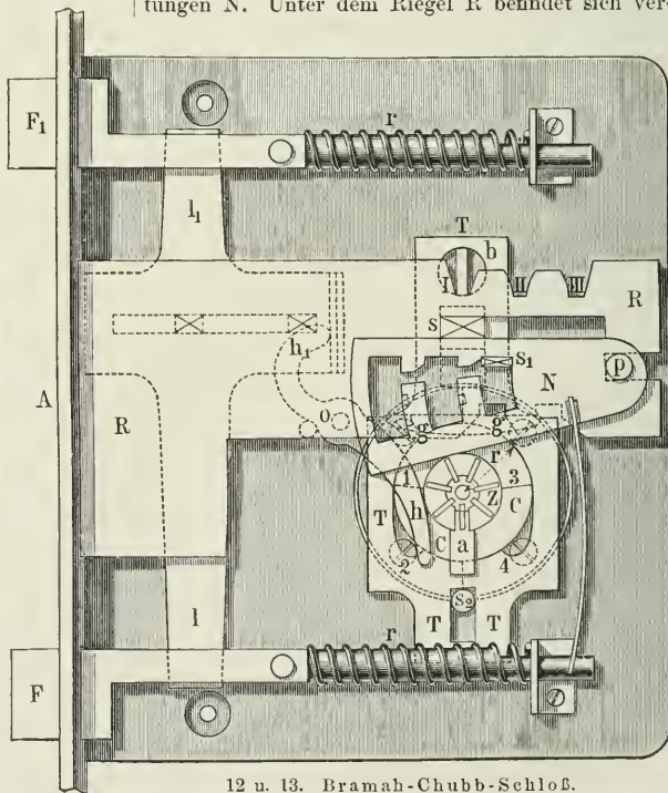
12 u. 13. Bramah-Chubb-Schloß.
