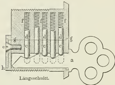
20. Yale-Schloß.
