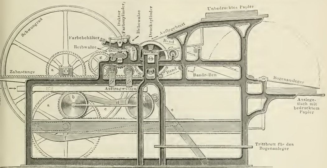
1. Ältere Schnellpresse mit Eisenbahnbewegung und einfachem zylindrischen Farbwerk (Ansicht).
