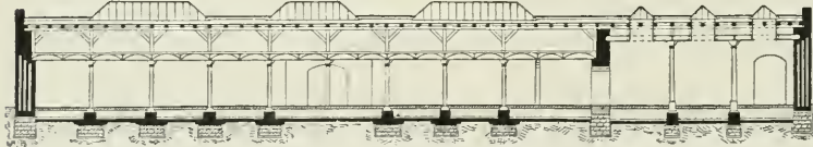
16. Kühlhaus. Längsschnitt.
