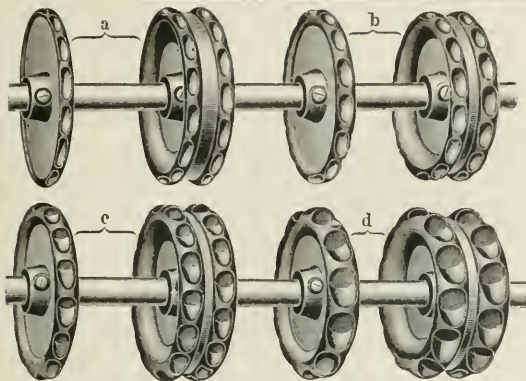
1. Auswechselbare Schöpfräder von Sack, Leipzig-Plagwitz.
