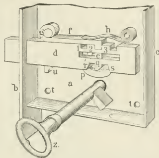
3. Französisches Schloß.
