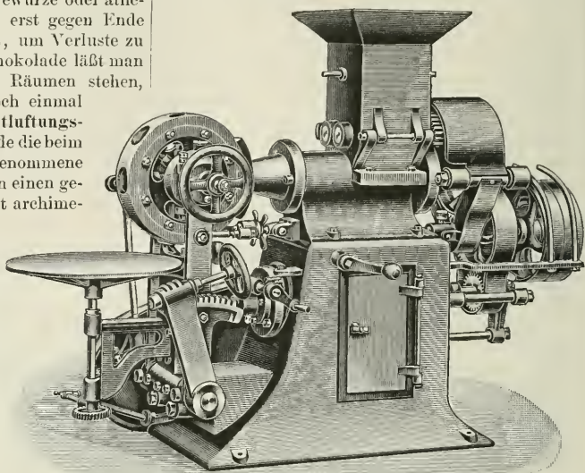
6. Entluftungsmaschine.
