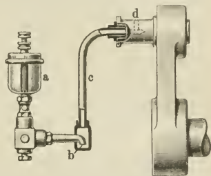
Fig. 7. Kurbelzapfenschmierung.
