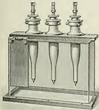
7. Dreiteiliger Wehnelunterbrecher.
