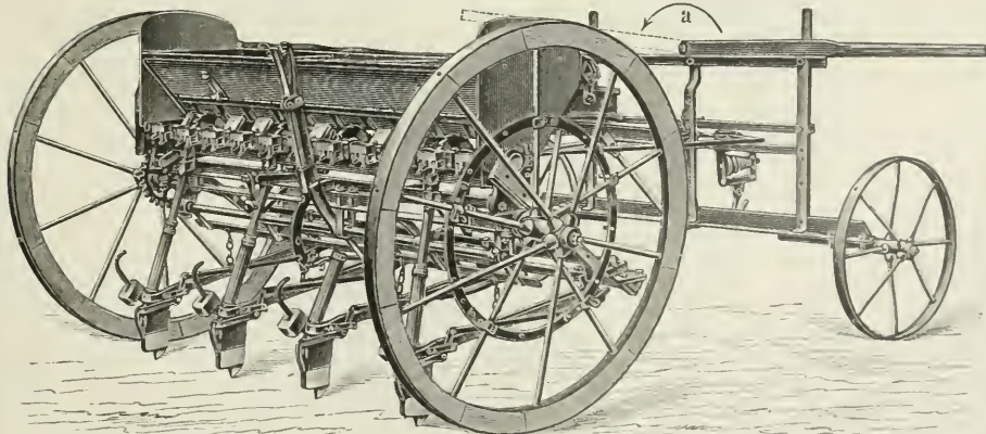
5. Drillmaschine Klasse I, vierreihig, mit Klappdibbelapparat, für Rübenkerne, von Sack, Leipzig-Plagwitz.
