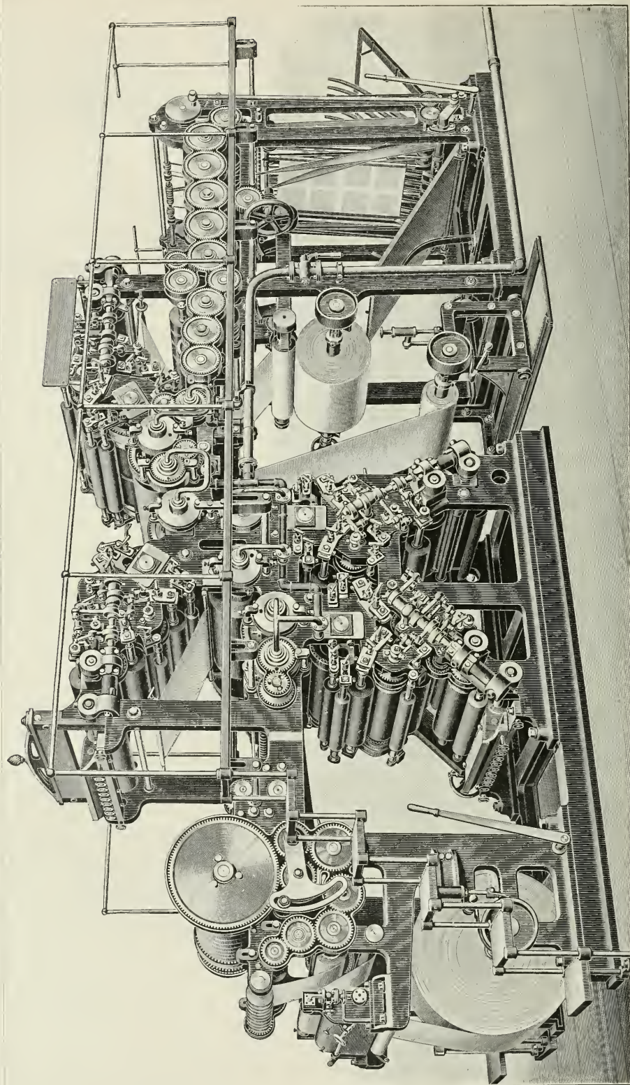
Zweifarb- Rotationsdruckmaschine für veränderliche Formate. Maschinenfabrik Augsburg.
