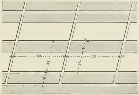
1 und 2. Abbau im Erfurter Steinsalzbergwerk.
