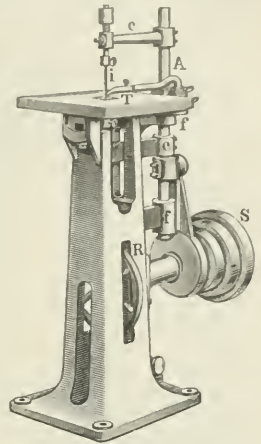
5. Säge- und Feilmaschine.
