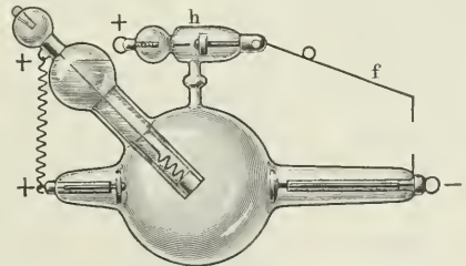
9. Müllerröhre mit Wasserkühlung und automatischer Selbstregulierung.
