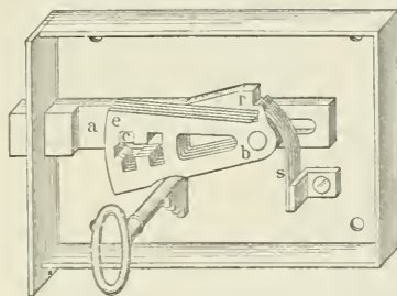
4—6. Chubb-Schloß.
