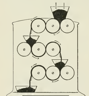
5. Schema einer Zylinderwalzmaschine.
