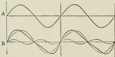
Fig. 2. Schwingungsformen.
