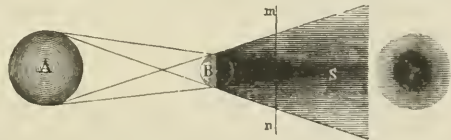
Fig. 2. Kern- und Halbschatten.
