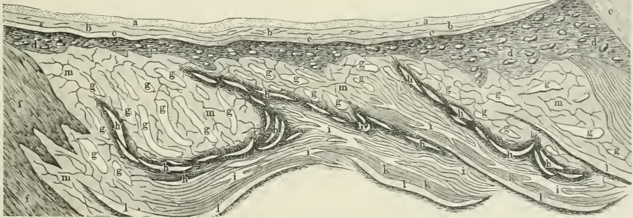
3. Querschnitt durch das Salzgebirge von Wieliczka.
