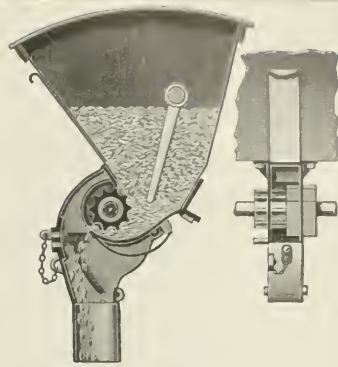
2. Schubradgehäuse von Eckert, Berlin.
