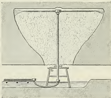
6. Steinsalzabbau durch Aussolung in Schönebeck.
