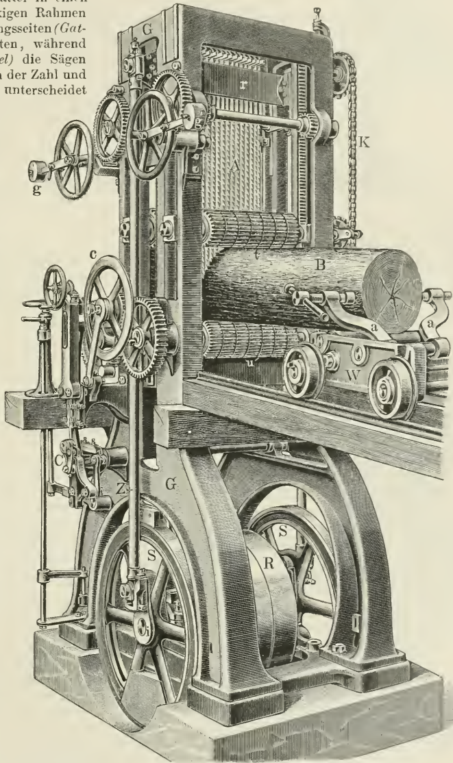
1. Vertikalvollgattersäge von Kirchner.
