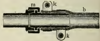
Fig. 6. Schlauchverbindung.
