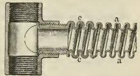
Fig. 7. Biegsames Metallrohr.
