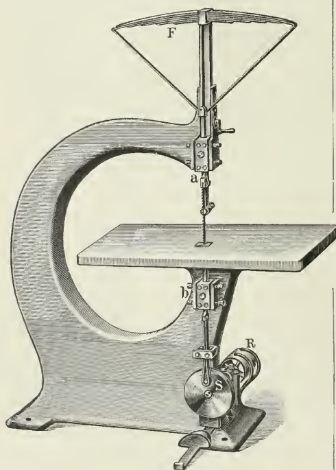
3. Wippsäge.
