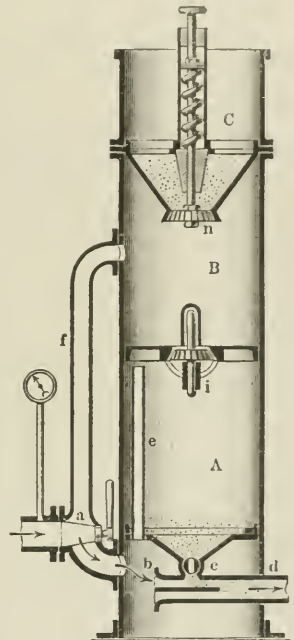
Drucksandstrahlgebläse von Gutmann.
