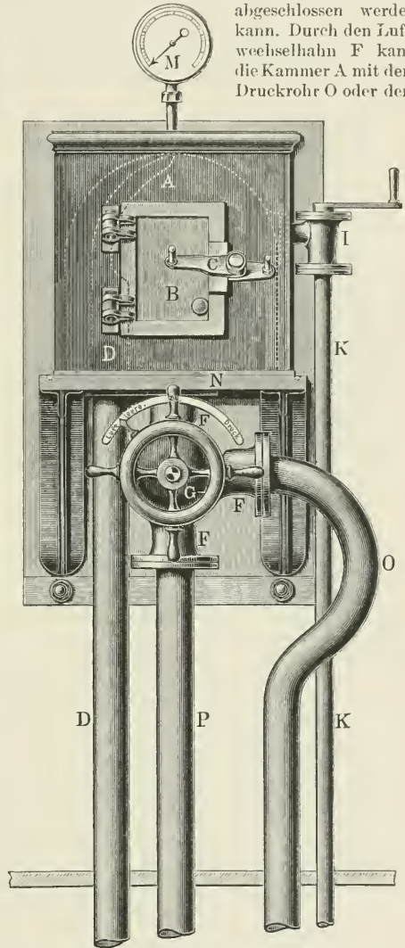
2. Rohrpostapparat. Endapparat mit Luftwechselhahn.
