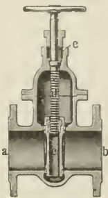
Abperrschieber.
