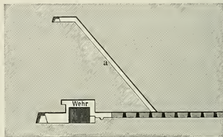
4 und 5. Vorrichtung zum Sinkwerksbetrieb in Berchtesgaden.
