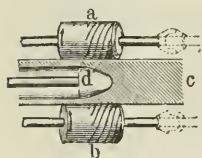
Fig. 3. Schrägwalzwerk.
