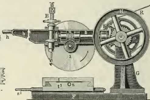
11. Kaltsäge.
