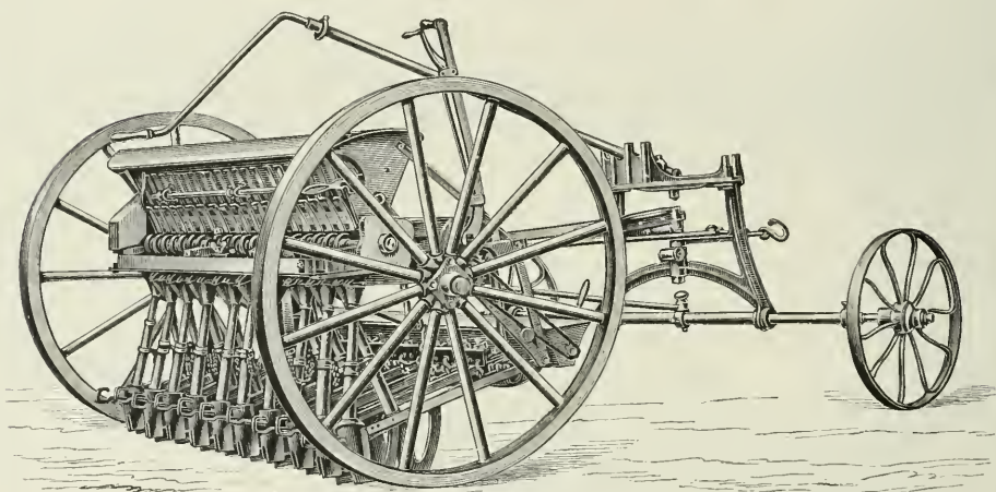
2. Nutenwalzen-Drillmaschine 'Berolina', mit Kleesäpparat, von Eckert, Berlin.
