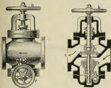
Ansicht. Rohrbruchventil. Durchschnitt.
