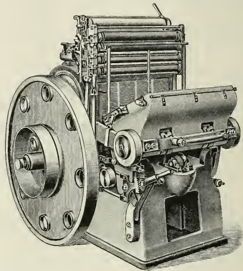
Akzidenzmaschine Victoria von Rockstroh u. Schneider Nachfolger in Dresden-Heidenau.
