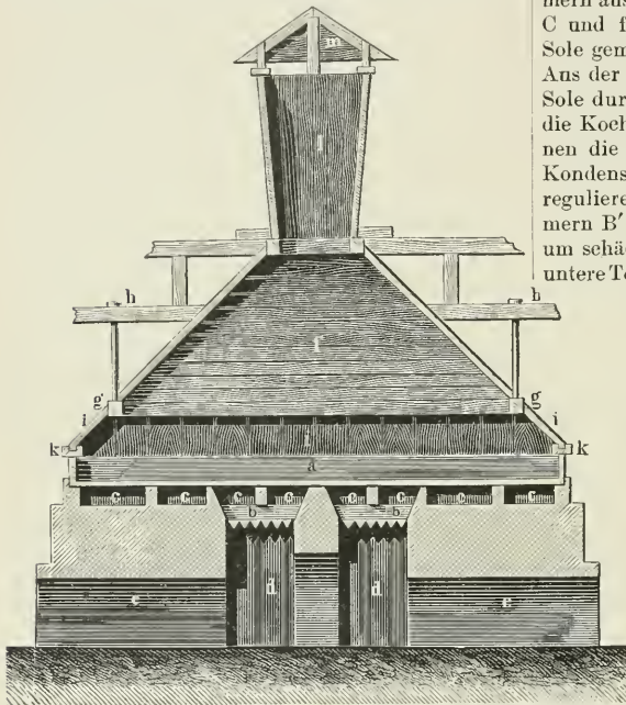
2. Siedevorrichtung mit Planrostfeuerung.
