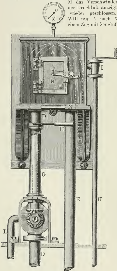
3. Zwischenapparat.
