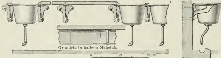
14. Kaldaunenwaschgefäße und Entfettungsplatten für Kuttelleien.
