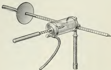
10. Funkenstrecke zur Unterdrückung der Schließungsströme.
