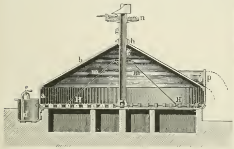
4. Rundpfanne mit Rührwerk.
