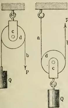
1. Feste Rolle. 2. Lose Rolle.
