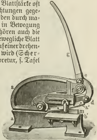
Fig. 1. Handhebelchere.
