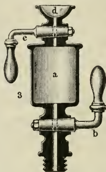
Fig. 3. Schmierhahn. Fig. 4. Kontinuierlich wirkender Schmierapparat.
