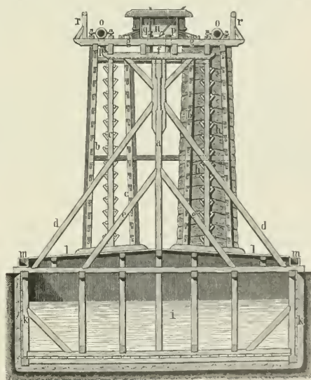
1. Dorngradierhaus.
