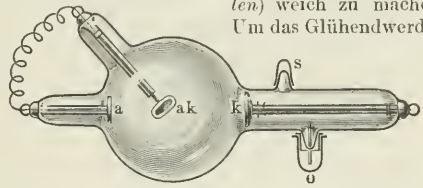
8. Einfache Röntgenröhre mit Osmoseregulierung.
