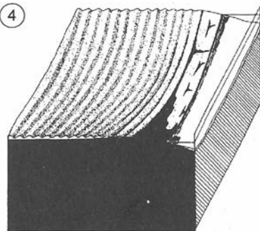
4 Anoxisches, schwarzes Porenwasser tritt am Prielhang oder aus Algenhaufen aus und bewirkt erhöhte Sauerstoffzehrung an der Oberfläche.
