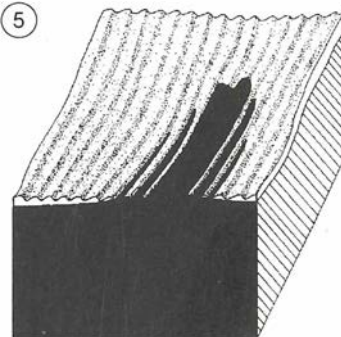
5 Der Redoxhorizont steigt aufgrund erhöhter Mineralisation an. Die oxische Sedimentschicht wird dünner und verschwindet schließlich völlig.
