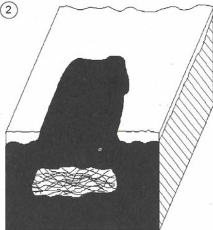
2 Makroalgen werden in das Sediment eingearbeitet und anaerob abgebaut. Das reduzierte, schwarze Sediment durchbricht die oxische Schicht an der Oberfläche. In der Tiefe kann es zur Bildung von überwiegend methanhaltigen Gasen kommen.
