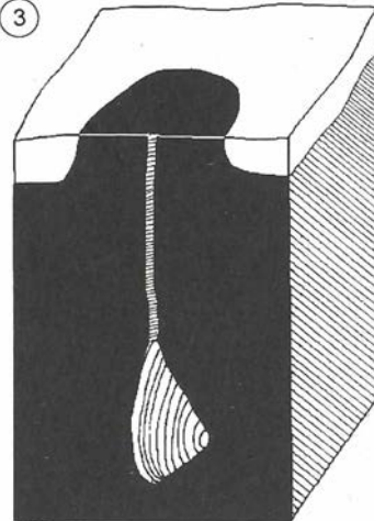
3 Endobenthische Organismen, z.B. Mya arenaria sterben ab und werden abgebaut. An der Oberfläche entsteht ein kleiner schwarzer Fleck.
