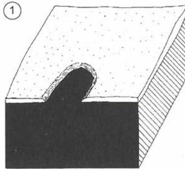
1 Erosion entfernt das oxische Sediment und legt so das schwarze Sediment frei. Das Phänomen tritt sowohl auf Wattflächen (Skizze) als auch im Verlauf von Prielien auf.
