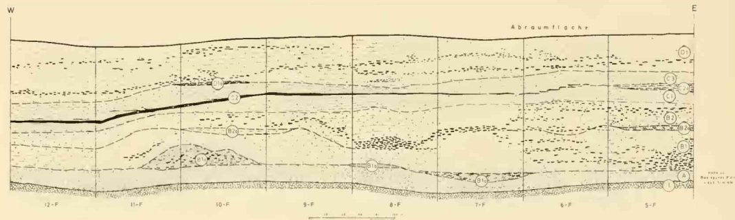
Abb. 8: Geologisches Profil der F-Schicht an der Nordwand der Planquadrate 5-F bis 12-F im Bereich der Grabungsstelle Ost (vgl. Abb. 5—6) in der Kiesgrube KARBER in Sandelzhausen. Erläuterungen der Schichtbezeichnungen im Text.
