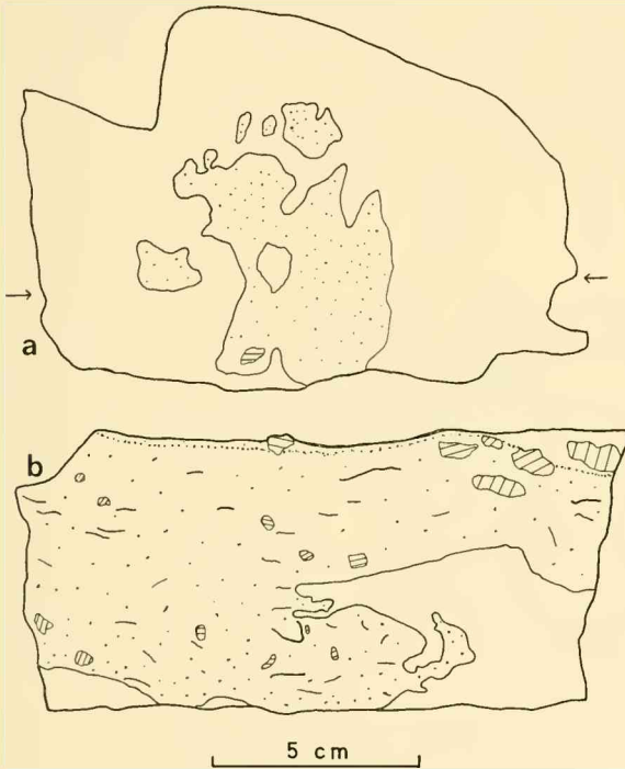
Abb. 1: Sedimentsstruktur in den Plattenkalken von Hennhüll, Steinbruch HARTEIS. Eine detritische Lage greift stellenweise in die liegende mikritische Schicht hinein. a) Aufsicht auf die Schichtunterseite, b) Vertikalschnitt (parallel der in a durch die Pfeile markierten Linie). Punktiert: detritisch; weiß: mikritisch; schraffiert: größere Fossilreste.
