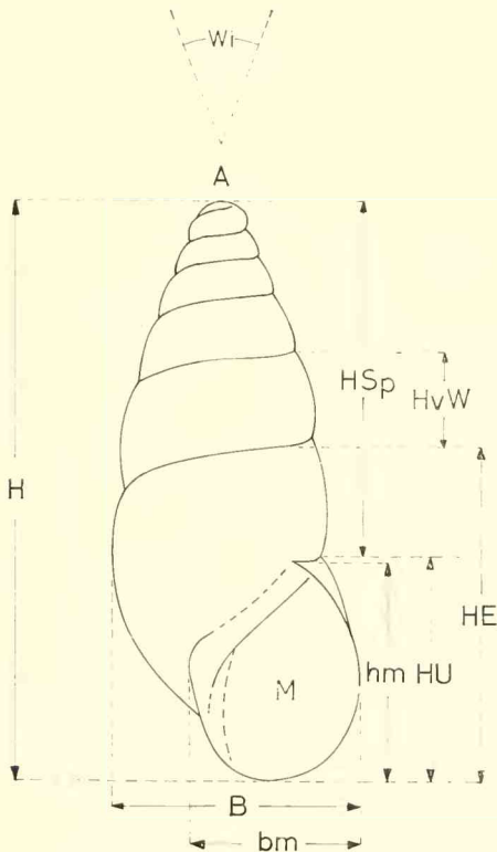
Abb. 1: Morphologie eines Gastropodengehäuses — Darstellung wichtiger terminologischer Einzelheiten.
