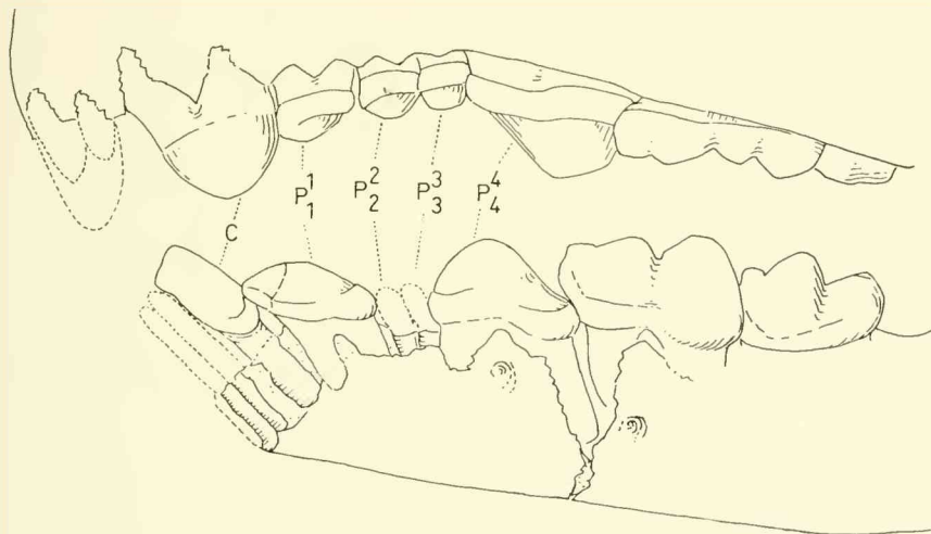
Abb. 10: Das Gebiß von Dimyloides stehlini HÜRZELER. — Die Oberkieferbezahnung ist die des Schädelfragments 1971 XXV 96 (vgl. Abb. 1a und Taf. 5, Fig. 1). Die Unterkieferbezahnung wurde durch die Kombination von zwei Mandibelfragmenten und zwei Einzelzähnen von Ehrenstein 4 rekonstruiert: es sind der linke Unterkieferrest mit P_1 und P_4 1971 XXV 94 (vgl. Abb. 2), das linke Unterkieferfragment mit M_2 1971 XXV 90, der linke M_1 1971 XXV 86 und der linke untere Eckzahn 1971 XXV 93. 9-fach vergrößert.
