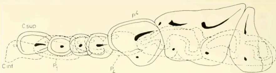
Abb. 7: Gebißokklusion von Plesiodimylus chantrei GAILLARD. Sie zeigt die einzige Möglichkeit des Ineinandergreifens von Ober- und Unterkieferzähnen bei geschlossenem Gebiß. Der von HÜRZELER (1944, S. 13) als unterer Canin (C inf.) angesprochene Zahn wird hier als erster Prämolare ( P_1 ) interpretiert. Die Oberkieferzähne (durchgezogene Linien) sind nach A. MÜLLER 1967, Abb. 9, die Unterkieferzähne (gestrichelte Linien) sind nach A. MÜLLER 1967, Abb. 10, in gleichem Maßstab umgezeichnet. 13-fach vergrößert.
