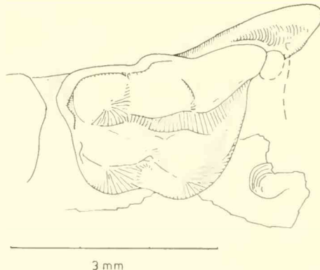
Abb. 4: Linkes Oberkieferfragment von Plesiodimylus chantrei GAILLARD aus La Grive-St.-Alban, 1965 I 144, von occlusal gesehen (Teilansicht) mit dem freien Ende des Maxillarfortsatzes.
