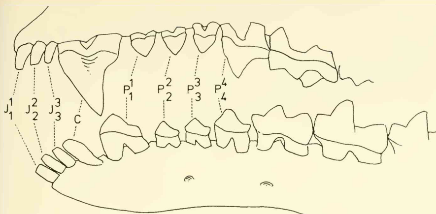
Abb. 9: Das Vordergebiß von Talpa europaea LINNAEUS in der Seitenansicht. 9-fach vergrößert.
