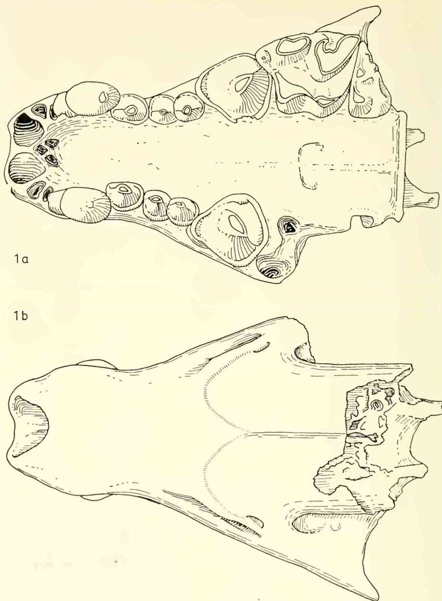
Abb. 1: Vorderschädel von Dimyloides steblii HÜRZELER aus der oberoligozänen Spaltenfüllung Ehrenstein 4, 1971 XXV 96. 1a: von occlusal gesehen, 1b: von oben gesehen. Der Jochbogen ist nicht abgebrochen, sondern fehlt primär. 8-fach vergrößert.
