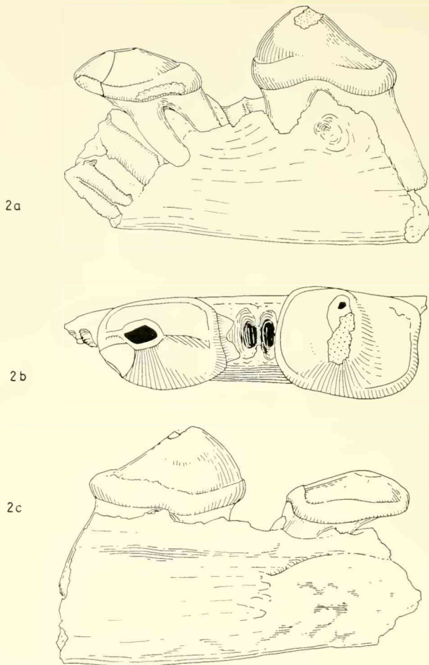
Abb. 2: Linkes Unterkieferfragment von Dimyloides steblini aus Ehrenstein 4 mit P_1 und P_4 und den Alveolen von P_2 , P_3 , C und den beiden Incisiven, 1971 XXV 94. 2a: von buccal, 2b: von occlusal, 2c: von lingual gesehen. 15-fach vergrößert.
