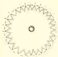
Abb. 2: Schematischer Querschnitt durch die Achse der Kaktsee Ferocactus wislizenii ; nach WALTER, Abb. 269 (verändert)
