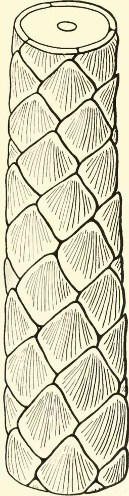
Abb. 1: Rekonstruktion eines Zweigstückes von Brachyphyllum nepos SAPORTA (in Anlehnung an Stück 1974 I 58, vergl. Taf. 3, links); ungefähr \times 3 (Zeichnung: H. THEILE)
