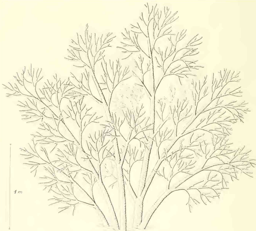
Abb. 3: Habitus-Rekonstruktion von Brachyphyllum nepos SAPORTA (Zeichnung: H. THIELI)
