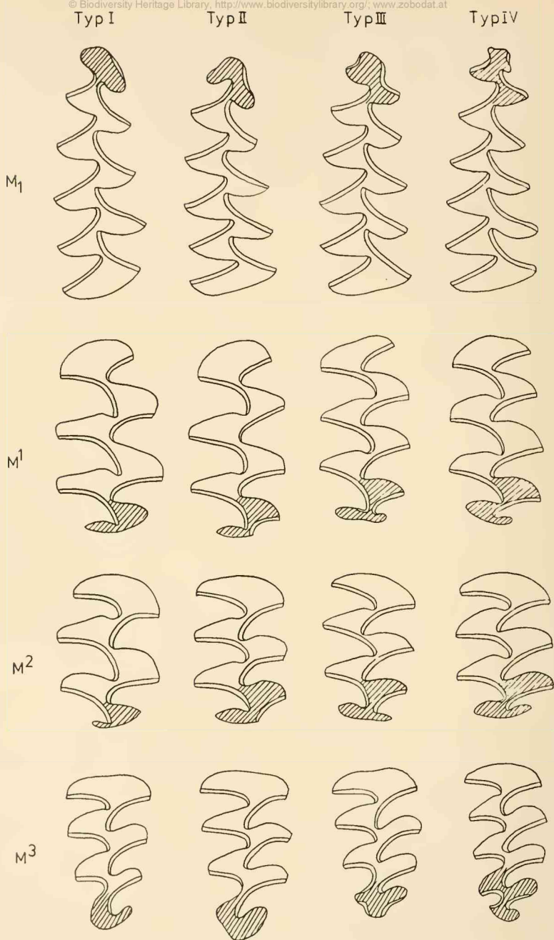
Abb. 3: Die wichtigsten Zahnmorphotypen von Dicrostonyx in der zweiten Hälfte des Pleistozäns.
