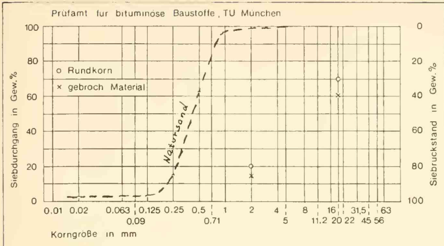
Abb. 9: Körnungskurve der aeolischen Talsande bei Illing II.
