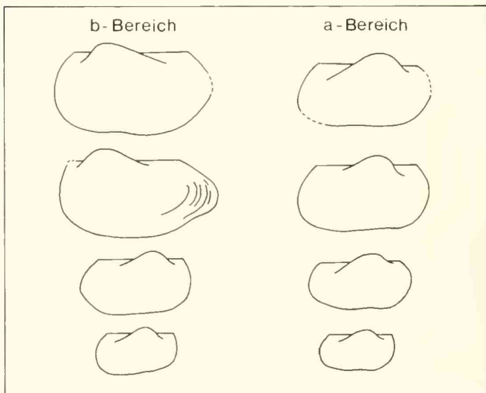
Abb. 2: Barbatia (Barbatia) ubligi (BOEHM). (oben): Die Variation des Umrisses und Übergang des Dorsalrandes in den Vorder- und Hinterrand. – (unten): Ein Vergleich des Umrisses der Kurzformen aus dem b-Bereich und der Langformen aus dem a-Bereich. AD = Anterodorsal; PD = Postero-dorsal.
