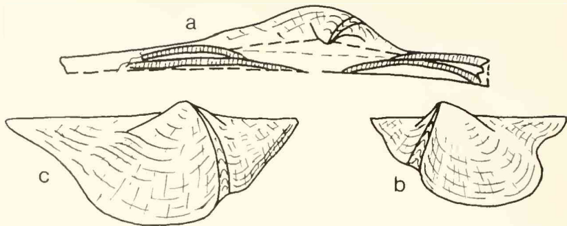
Abb. 3: Stenocolpus biburgensis n. gen. n. sp. a) Schematische Darstellung des Schlosses und der Ligament-Area aus der Kombination von zwei Exemplaren (1980 XXX 2–3). – b) Umriß des Holotyps: 1980 XXX 1. X 1,5, Kurzform. – c) Umriß des Paratypes: 1980 XXX 5. X 1,5, Langform.
