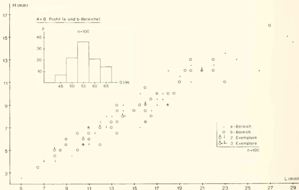
Abb. 1: Barbatia (Barbatia) uhligi (BOEHM). Längen-/Höhenverhältnis von 100 Exemplaren aus dem a- und b-Bereich des Profils. – (oben): Verteilung des Diameterindex derselben Exemplare.
