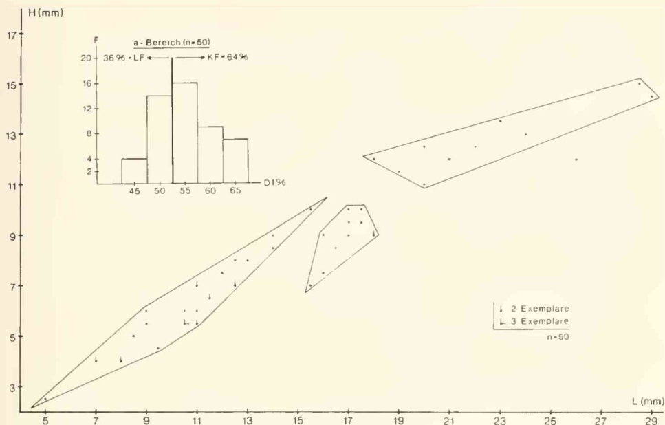
Abb. 5: Barbatia (Barbatia) uhligi (BOEHM). Längen-/Höhenverhältnis von 50 Exemplaren aus dem a-Bereich des Profils. (Oben): Die Verteilung des Diameterindexes derselben Exemplare, die hier einen höheren Anteil an Langformen aufweist, als im b-Bereich.
