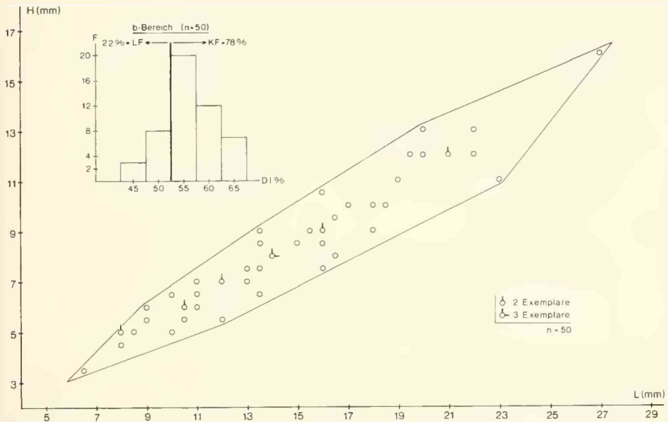
Abb. 4: Barbatia (Barbatia) uhligi (BOEHM). Längen-/Höhenverhältnis von 50 Exemplaren aus dem b-Bereich des Profils. (oben): Die Verteilung des Diameterindex derselben Exemplare, die eine Verschiebung zugunsten der Kurzformen (KF) im b-Bereich zeigt.
