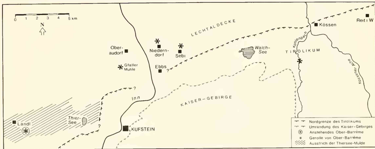
Abb. 4: Geologisch-topographische Fundortskizze der Urgonkalke SE Landl (Stern mit Kreis) und der Geröllvorkommen (Stern).
