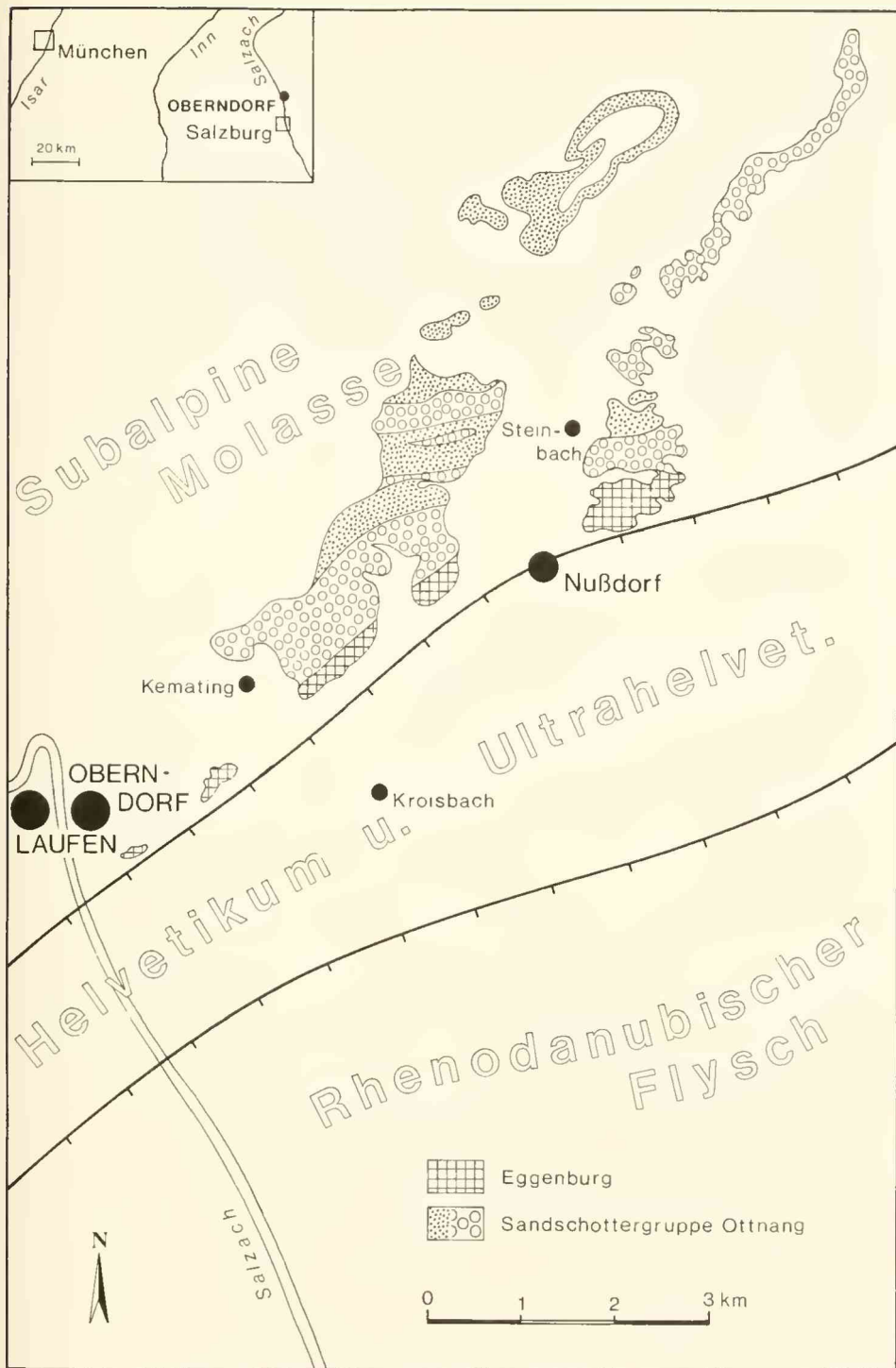
Abb. 1: Topographisch-geologische Übersichtsskizze.
