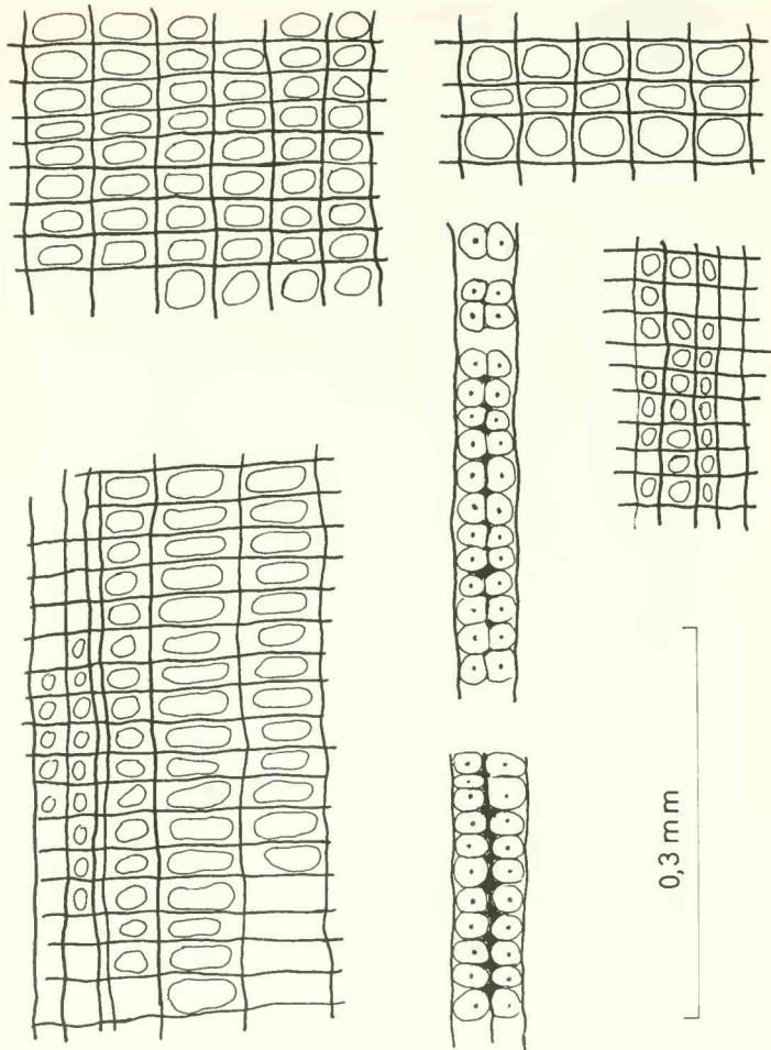
Abb. 4: Radialschliff. Kreuzungsfeld-Tüpfel im Früh- und Spätholz, vertikale Reihen teils gegenseitig abgeplatteter Tracheidenhoftüpfel. 1969 1 72.
