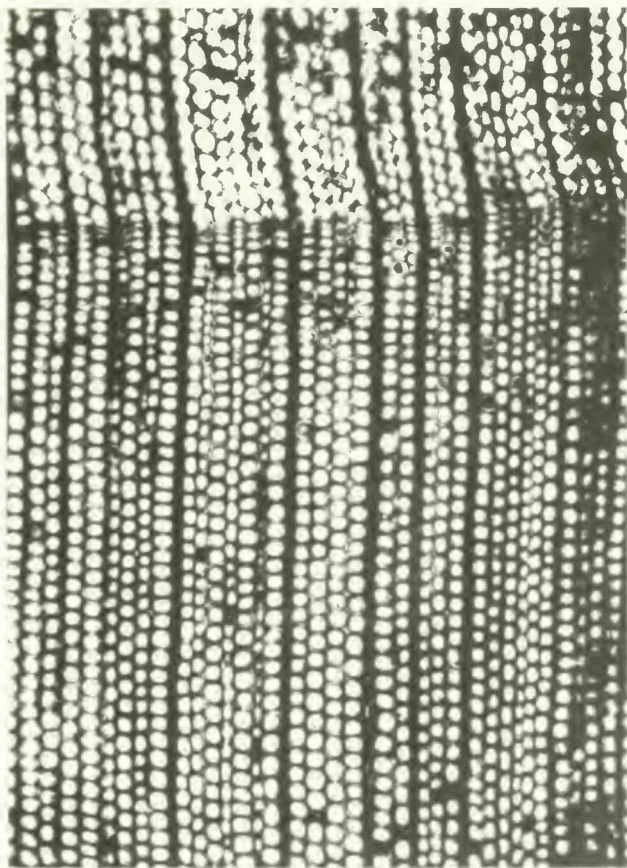
Abb. 1: Querschliff. Zuwachsgrenze, radiale Tracheidenreihen, dunkle Holzstrahlen, verstreute Parenchymzellen mit dunklem Inhalt. 1969 I 72; \times 40 .
