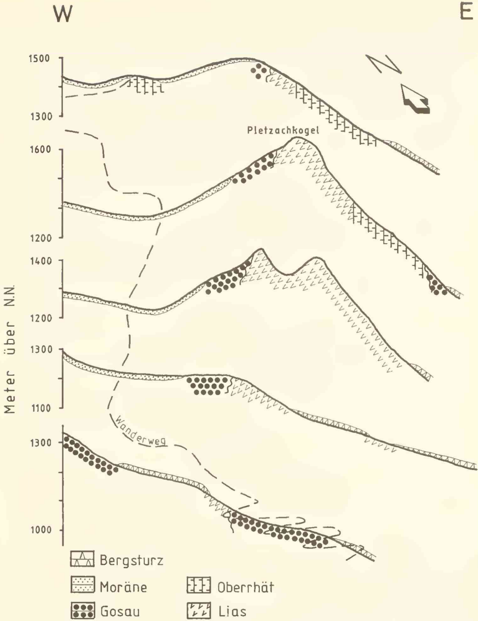
Abb. 3: Profilserie über den Pletzackkogel: Die steilstehenden Rhätoliaskalke am Pletzackkogel fallen mit 85° S zum Betrachter hin ein.
