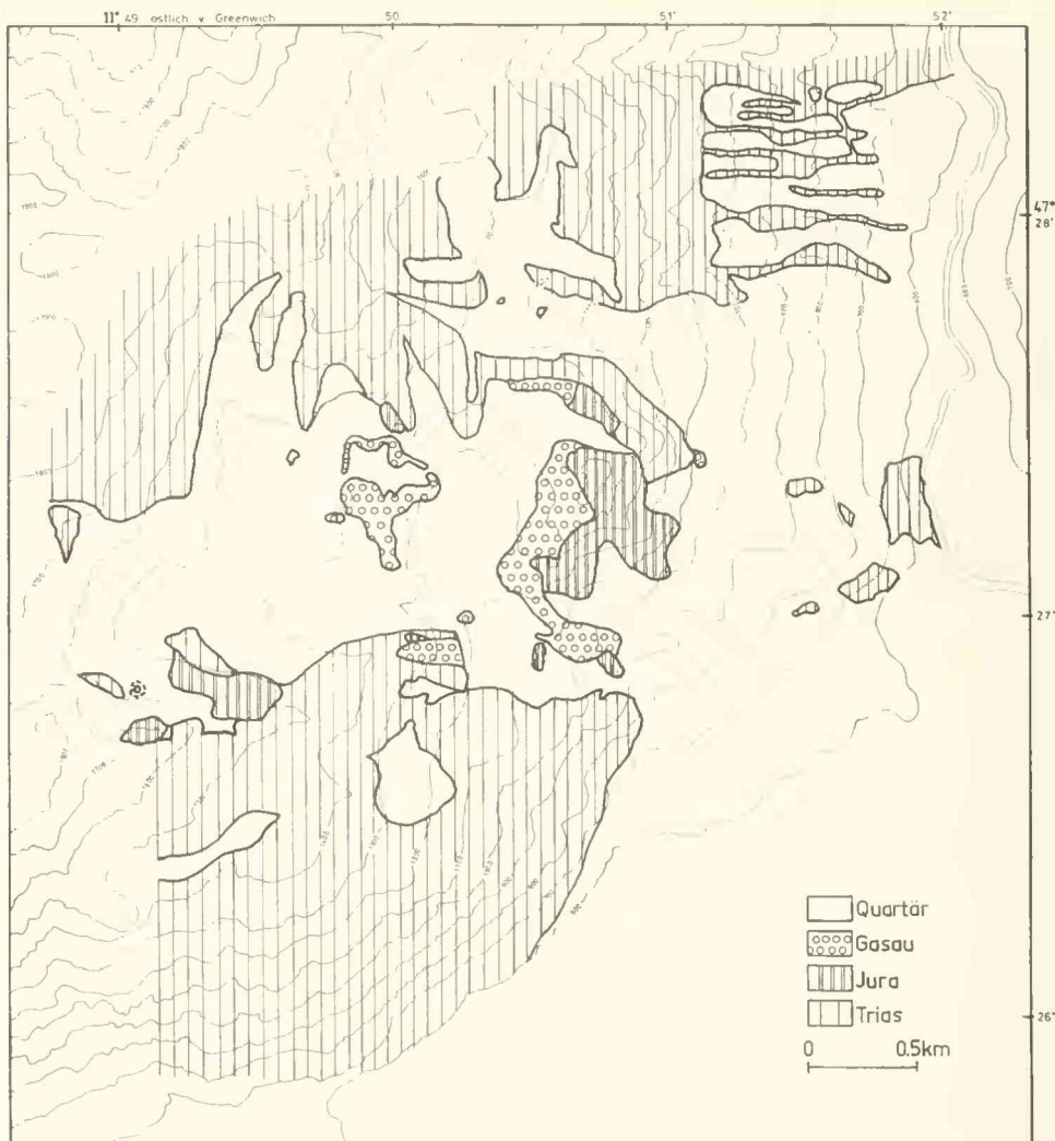
Abb. 1: Verbreitung der Gosau-Vorkommen im Raum Pletzachkogel, südöstliches Rofengebirge, Tirol
