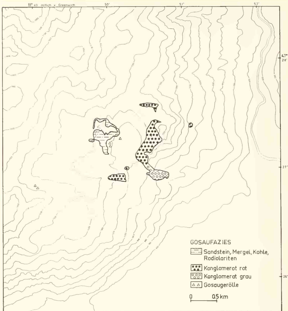
Abb. 2: Verbreitung der verschiedenen Faziesseinheiten in der Gosau am Pletzackkogel
