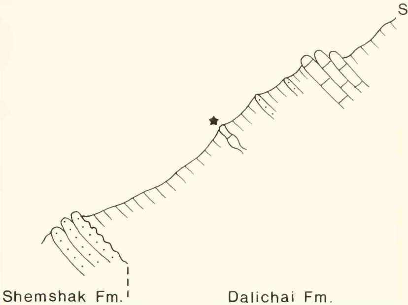
Abb. 5: Idealisiertes Profil der Dalichai-Formation am Nordabhang des Kuhe-Namord. *: Fossilfundpunkt.
