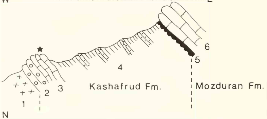
Abb. 3: Idealisertes Profil der Kashafrud-Formation bei Tappeh-Nader. 1: basische Vulkanite (?oberes Perm); 2: basales Konglomerat (ca. 5-6 m); 3: knollige, etwas sandige Kalke mit Ammoniten vor allem in den obersten Teilen (ca. 10 m); 4: viele hundert Meter dunkler, monotoner, z.T. turbiditischer Tonschiefer mit eingeschalteten sandigen Bereichen; 5: gelbroter Verwitterungshorizont (ca. 2 m); 6: rotlich-braune, oolitische, dickbankige Kalksteine (Mozduran-Formation), die mit deutlicher Diskordanz über der Kashafrud-Formation folgen. *: Fossilfundpunkt.
