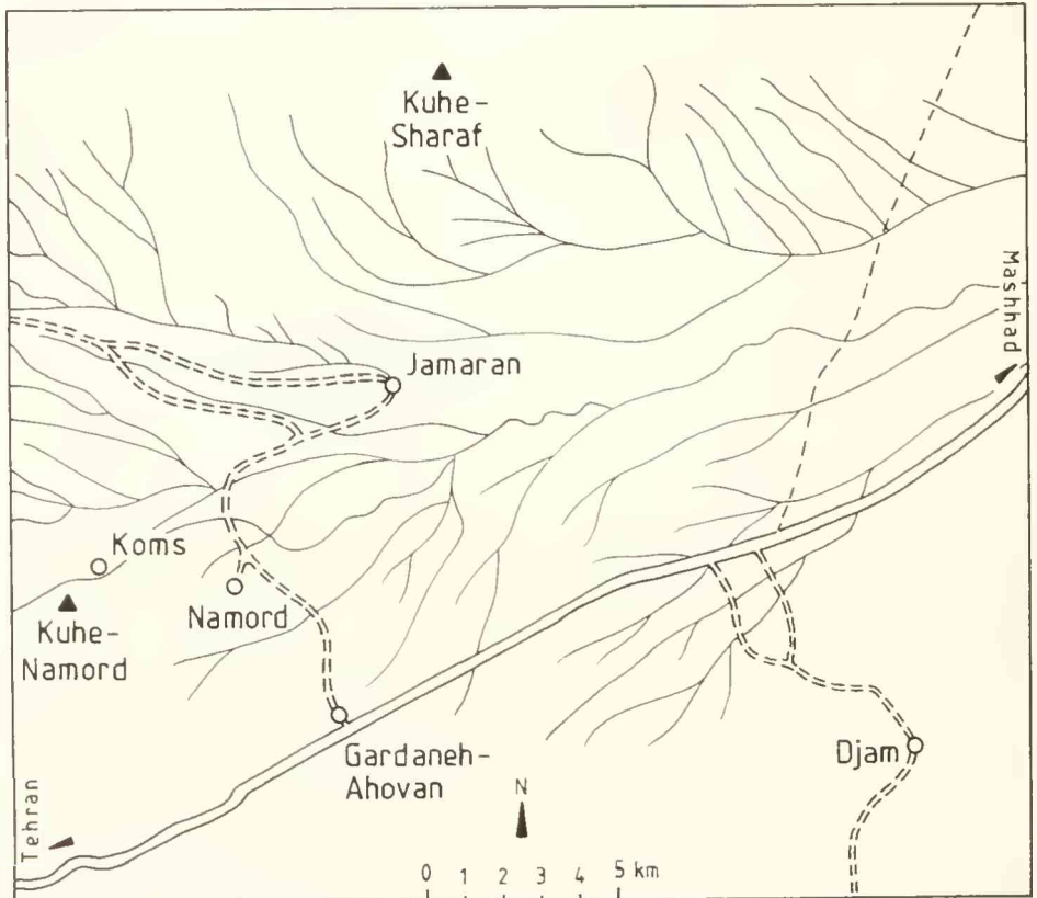
Abb. 4: Lageskizze von Kuhe-Namord und Kuhe-Sharaf im SE-Alborz.
