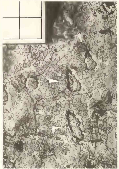
Abb. 3: vergrößerter Ausschnitt aus dem Gegenruck, drei Einzellogen aus einem Zickzackband, mittlere mit Eirest, jeweils mit stumpfem und spitzem Ende, Maßstab = 1 mm, Foto W. HELLMUND.
