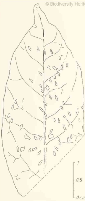
Abb. 1 a: Angiospermenblatt, (?) Juglandaceae, eine einzelne Fieder mit Eilogen vom „Coenagrioniden-Typ“, SMNS 62599, Randecker Maar (Baden-Württemberg), oberstes Untermiozän, Zeichnung M. HELLMUND.
