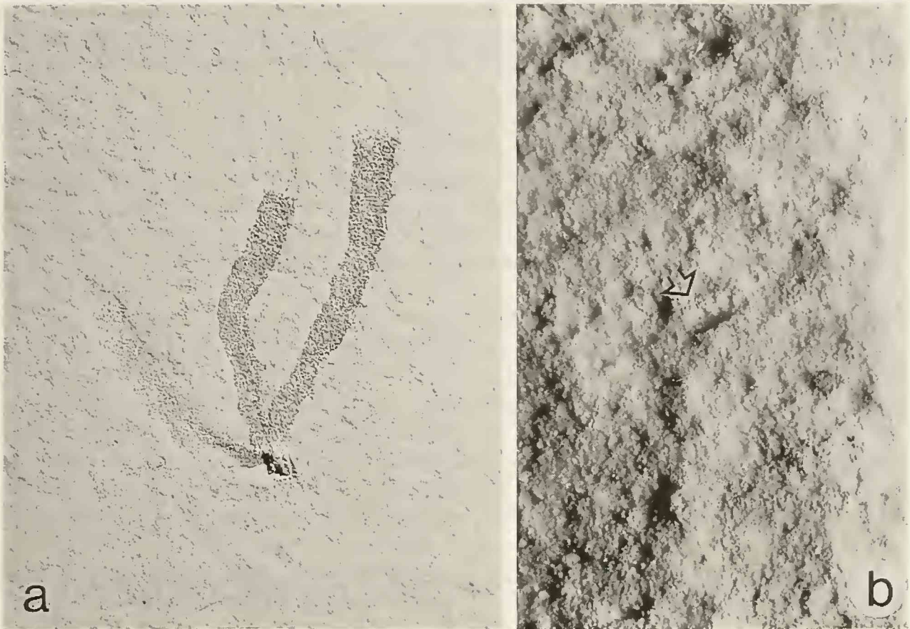
Abb. 1. a. Muensteria vermicularis STERNBERG. Solnhofener Plattenkalk, 3 auf einem Lithoklasten angeheftete Individuen. Unter-Tithonium, Hybonotum-Zone, Rueppellianum-Subzone, Langenaltheim. SMNS Inv.-Nr. 62828 (Coll. W. LUDWIG 1996). – nat. Größe. – b. Detail der Oberfläche von Muensteria vermicularis STERNBERG beim Holotypus von Epitrachys rugosus EHLERS (siehe Tafel 1, Fig. 1) mit agglutiniertes Foraminifere (Pfeil). – x 10.
