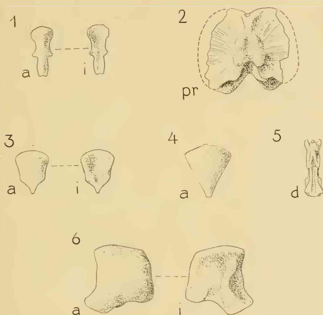
Abb. 1—6: Isolierte Ophiuren-Elemente aus den Neuburger Bankkalken (Mittel-Tithon) vom Bahnhof Unterhausen. \times 20 .
