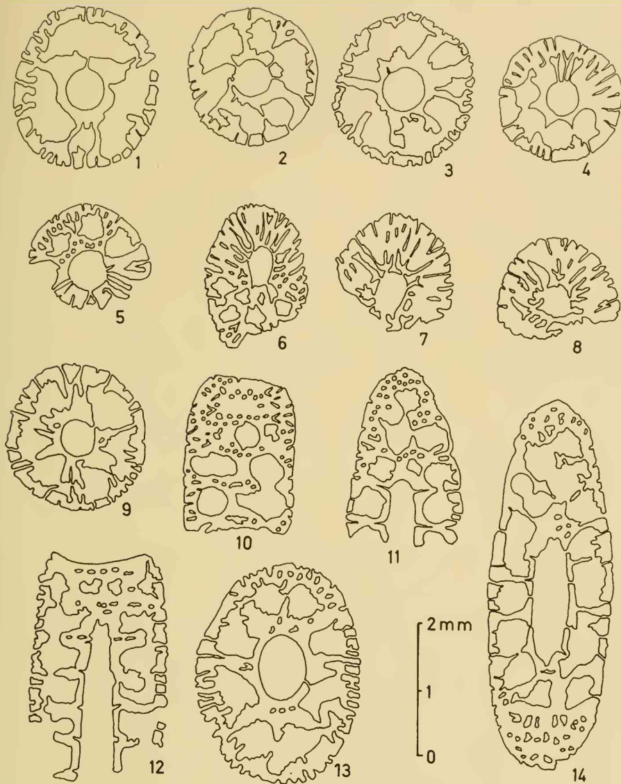
Abb. 5: Schnitte von Chinianella zankli n. sp.
