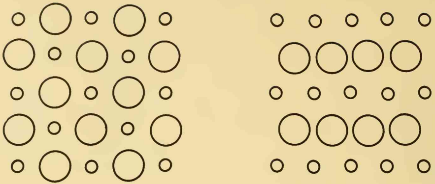
Abb. 2: Anordnung der sterilen Äste und der Sporangien (große Kreise) bei den Gattungen Cylindroporella JOHNSON (links) und Chinianella n. g. (rechts). Tangentiale Aufsicht, schematisch
