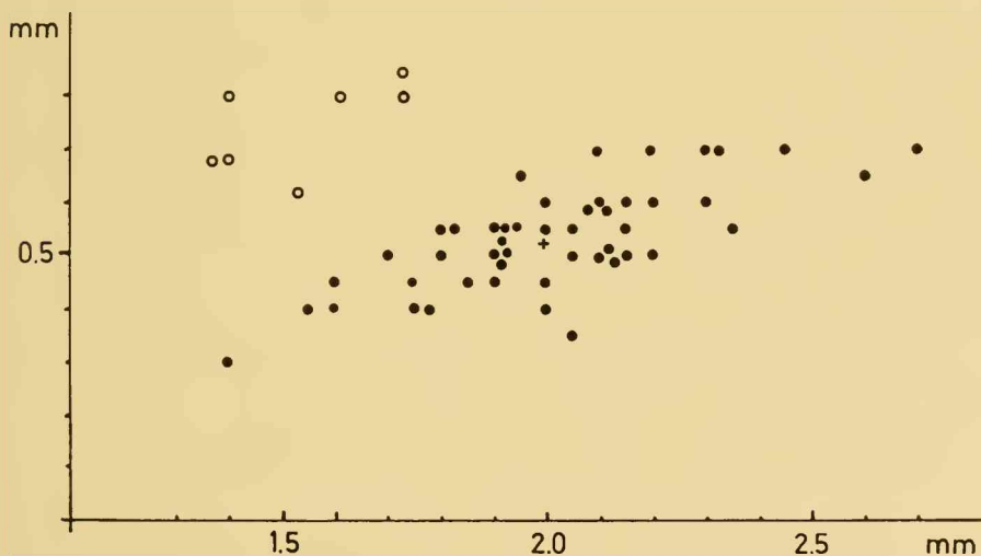
Abb. 4: Außendurchmesser/Innendurchmesser an 48 Exemplaren von Chinianella zankli n. sp. + = errechneter Mittelwert. — Kreise = Vergleichswerte von Chinianella ellenbergeri (LEBOUCHÉ & LEMOINE)
