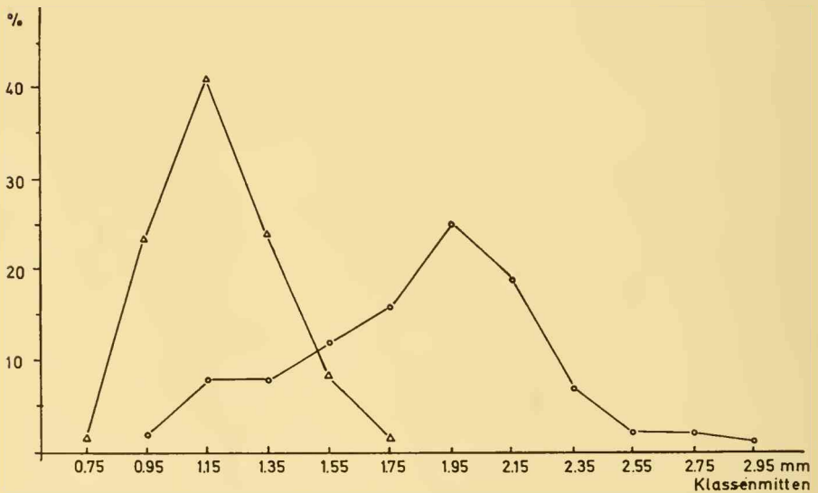
Abb. 1: Häufigkeitsverteilung des Außendurchmessers bei Diplopora tubispora n. sp. (linke Kurve, aus 241 Exemplaren) und Diplopora phanerospora P1A (rechte Kurve, aus 100 Exemplaren)
