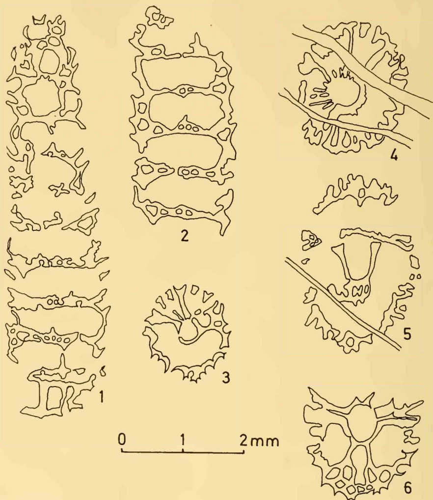
Abb. 3: Schnittbilder von Chinianella crosi n. sp.
