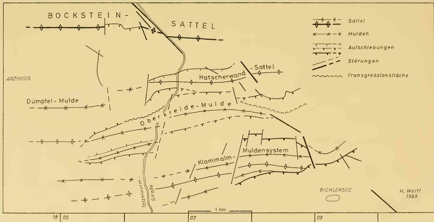
Abb. 3: Tektonische Übersichts-Skizze des östlichen Wendelstein-Gebietes zwischen Arzmoos und Bichler-See.
