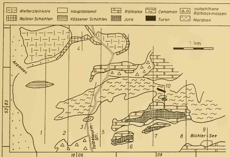
Abb. 1: Stratigraphische Übersichts-Skizze des östlichen Wendelstein-Gebietes zwischen Arzmoos und Bichler-See, mit Lageplan der auf Abb. 2 dargestellten Profile.
