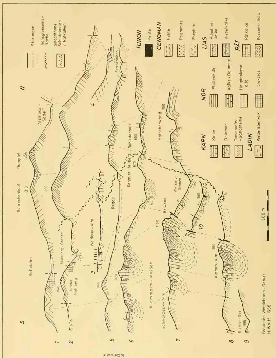
Abb. 2: Profil-Serie durch das östliche Wendelstein-Gebiet zwischen Arzmoos und Bichler-See.
