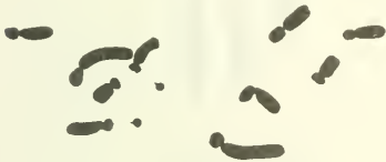
Abb. 1: Wurzelspitzen-Mitose von Crepis pusilla (= Melitella ); C. R. ALCOCK 1615, aus Samen gezogen im Bot. Garten München.
