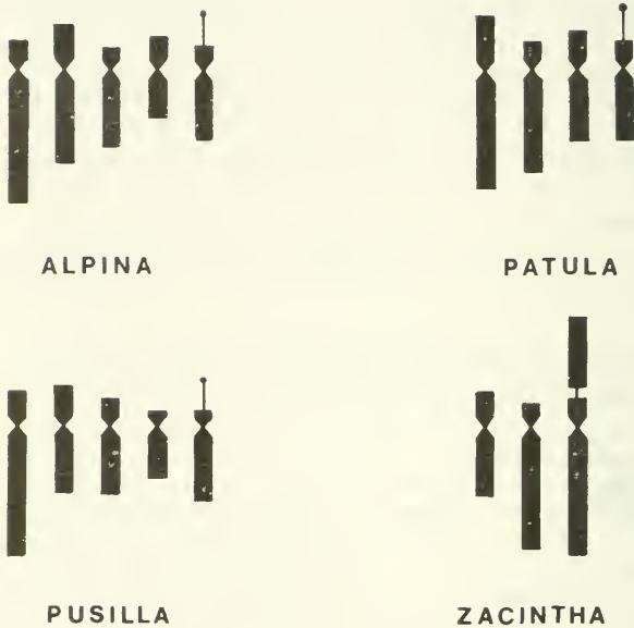
Abb. 2: Karyogramme von Crepis pusilla (= Melitella ), C. patula und C. zacinctha sowie von C. alpina .
