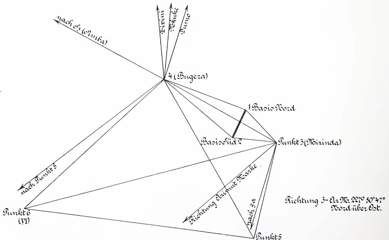
Skizze 4. Basis-Netz bei Nyangoma.
