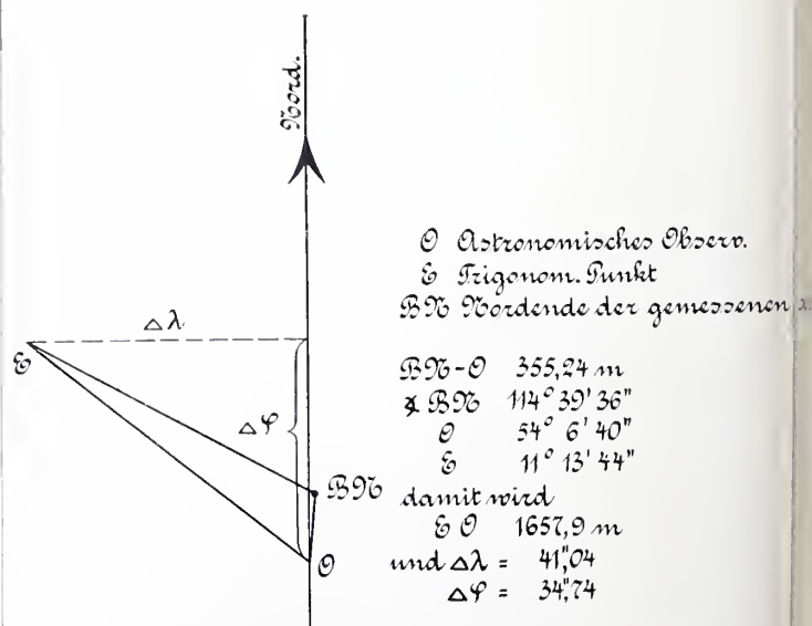
Skizze 3. Übertragung der Koordinaten in Entebbe.
