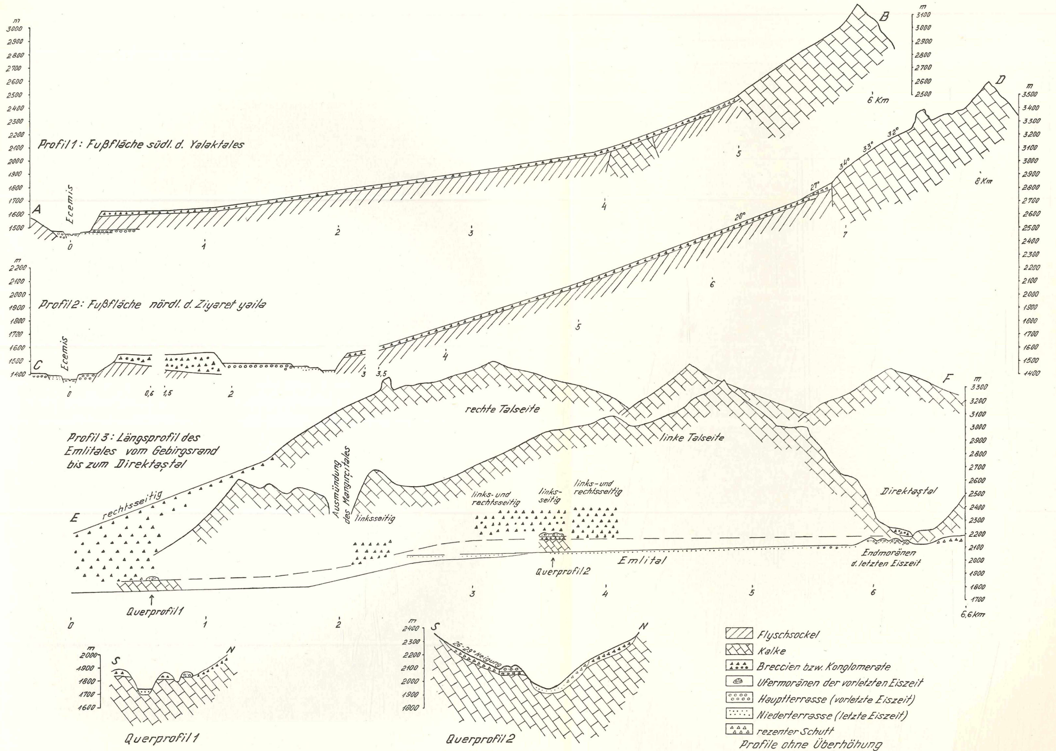
Zu Querprofil 2: Der Hang mit 26—29° Neigung ist von mächtiger alter Breccie (nicht von rezemem Schutt) eingenommen; die Breccie entspricht den Konglomeraten unter der Ufermoräne sowie auch der Breccie des gegenüberliegenden Hanges.
