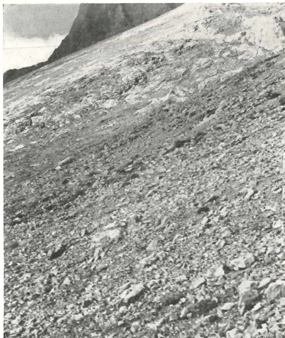
Bild 3. Glatthang an der Westseite des Ala Dag nördlich der Esnevitvayla von 2800 m an aufwärts; im Vordergrund Schuttbedeckung der untersten Partie des Glatthangs. Aufn. Spreitzer, 8. VIII. 1955
