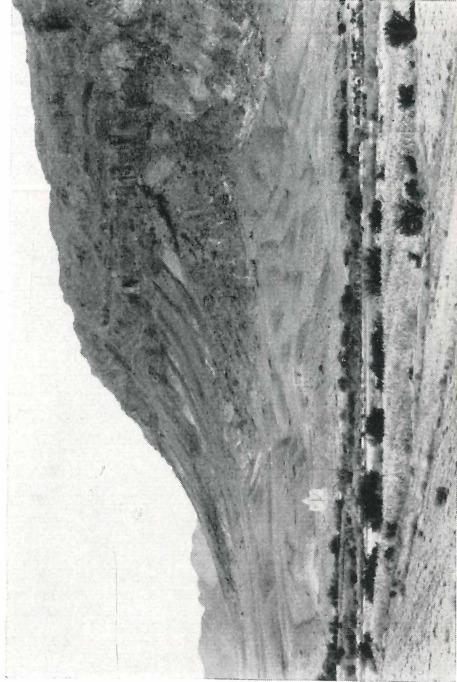
Bild 5. Steilhang in Jurakalken und -mergeln einer Kette im östl. Hohen Atlas. In halber Höhe ist der mit einer Breccie bedeckte Rest eines älteren Hanges erhalten geblieben, gegenüber dem der heutige durch Verwitterung, Massenbewegungen und Abspaltung nicht unerheblich zurückverlegt wurde. Phot. K. WICHE.
