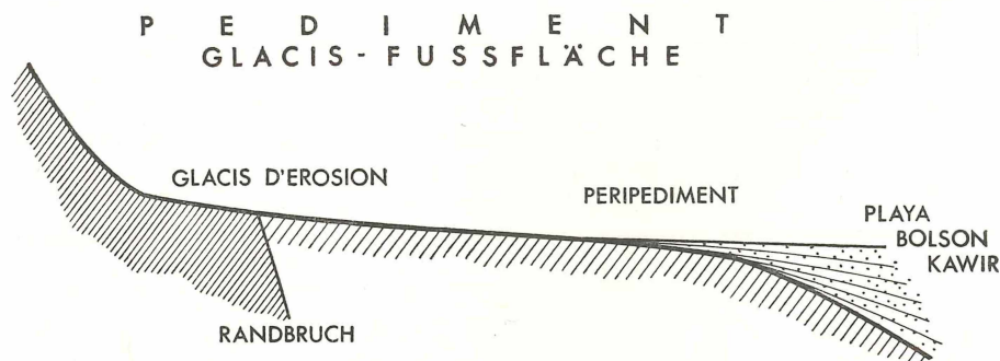
Abb. 1. Längsschnitt durch ein Pediment am Fuße eines tektonisch angelegten Steilhanges.
