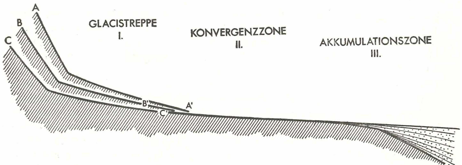
Abb. 2. Die Zonen eines mehrgliedrigen Pediments. Die Konvergenzzone stellt den polygenetischen Teil des Glacis dar.
