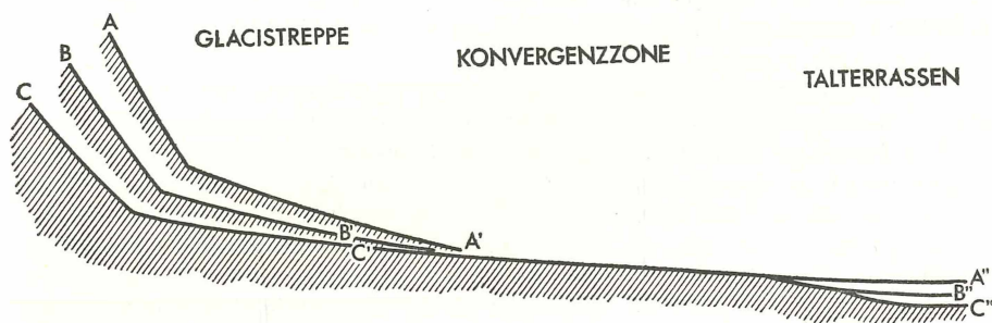
Abb. 3. Mehrgliedriges Pediment mit terrassiertem Einschnitt, der von einem stärkeren Gerinne in die Konvergenzzone zurückgreift.
