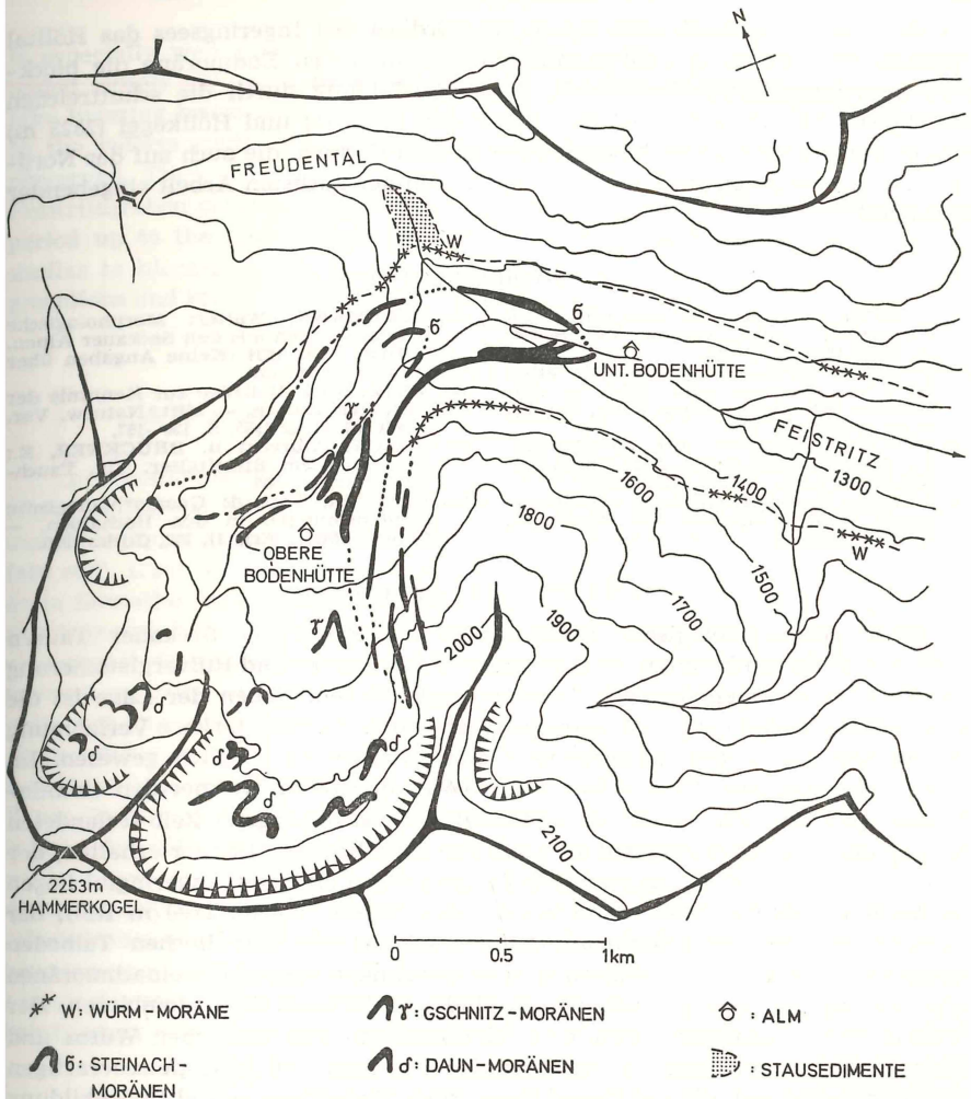
Abbildung 2 Moränen Oberes Feistritztal/Bodental (Entwurf H. NAGL)
