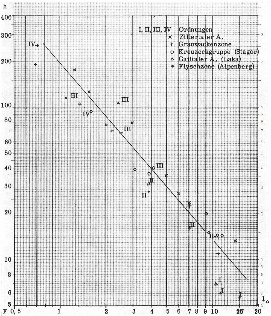
Abbildung 2: Streuungsdiagramm: Eintiefung — Flußhäufigkeit
