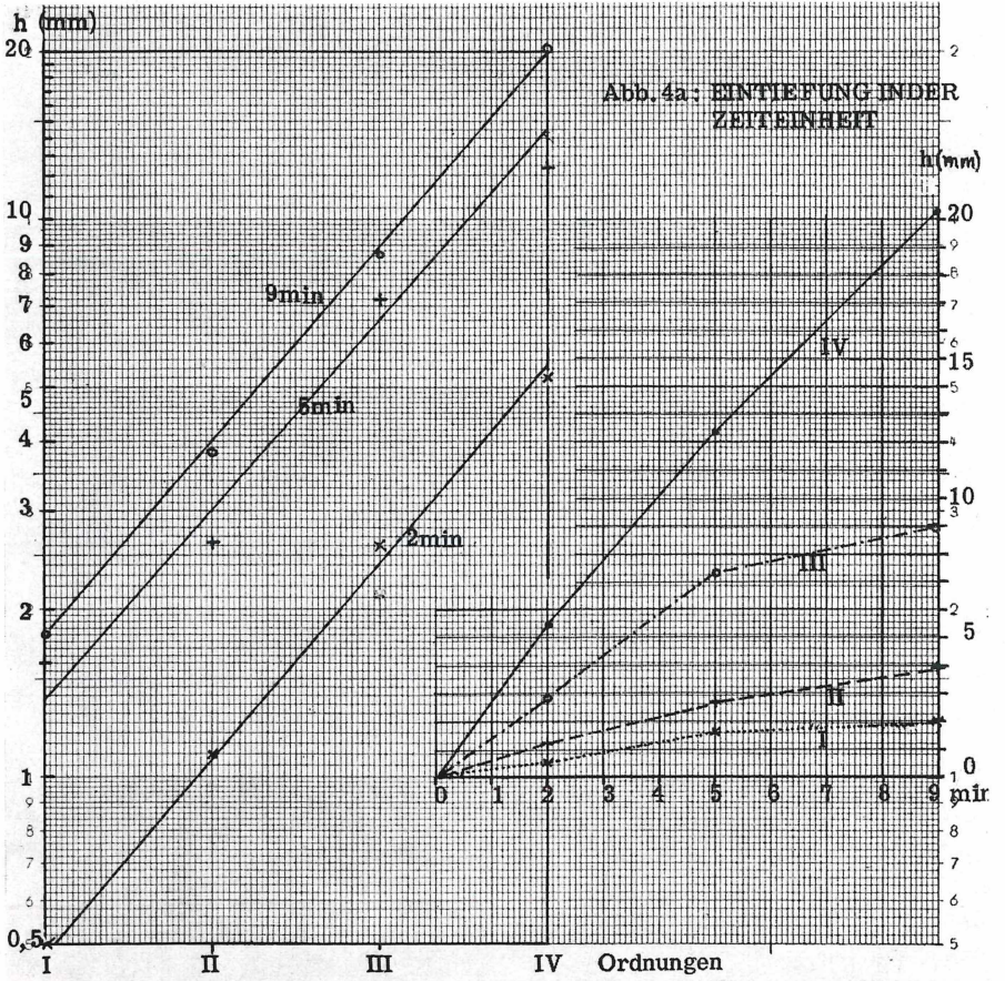
Abbildung 4: Eintiefungsverhältnis von Rinnensystemen im Laborversuch. Hangneigung 30^\circ
