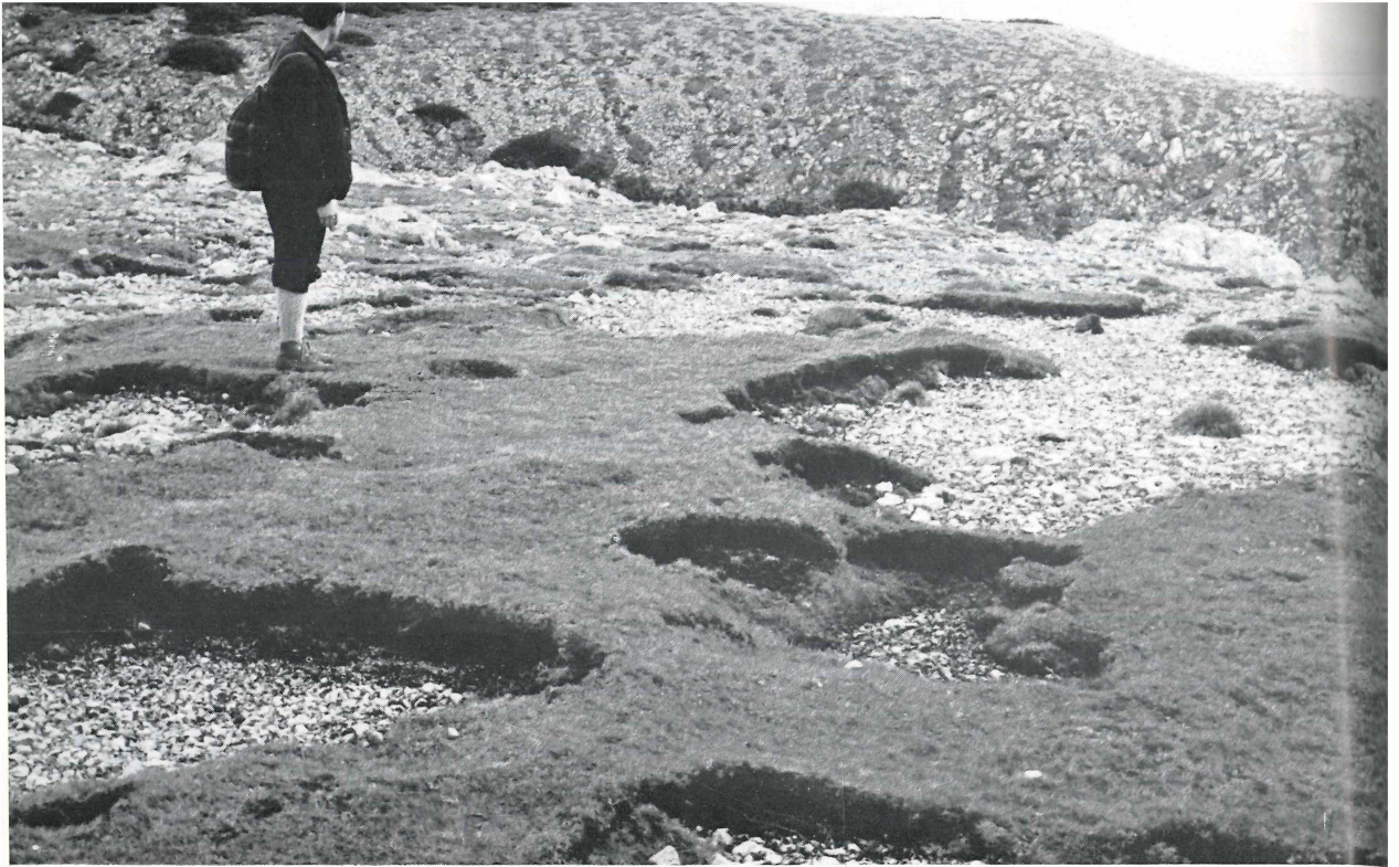
Bild 3: Rezente Rasenschälung (Raxalpe 1740 m)
