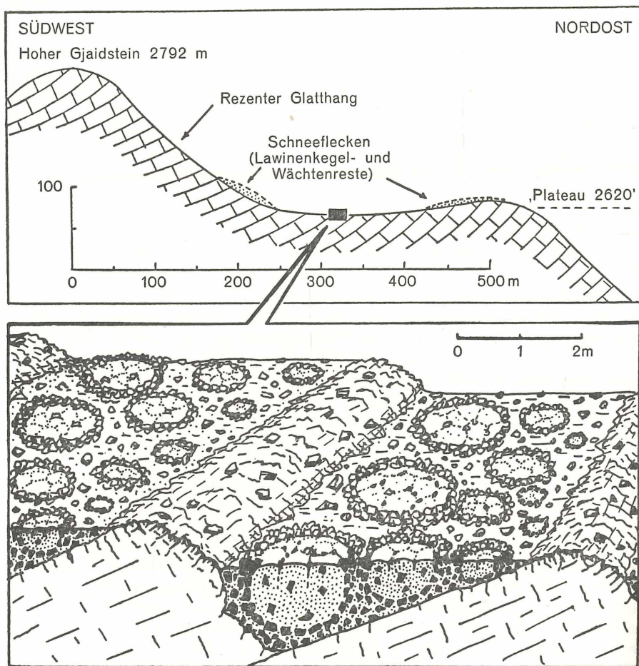
Fig. 10: Die Steinring-Großformen am Gjaidstein (Dachsteingebiet)
