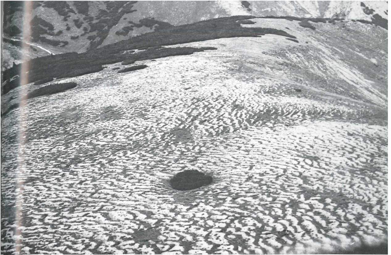
Bild 5: Rasengirlanden (Leegirlanden) im Dolomit (Schneealpe 1720 m)
