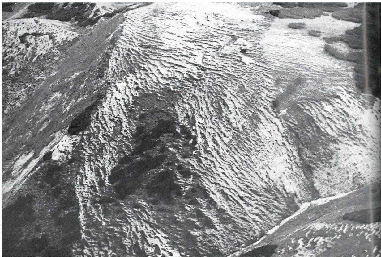
Bild 7: Diagonale Rasenstreifen (Diagonalgirlanden) bei tangierender Hauptwindrichtung (Schneealpe 1700 m)
