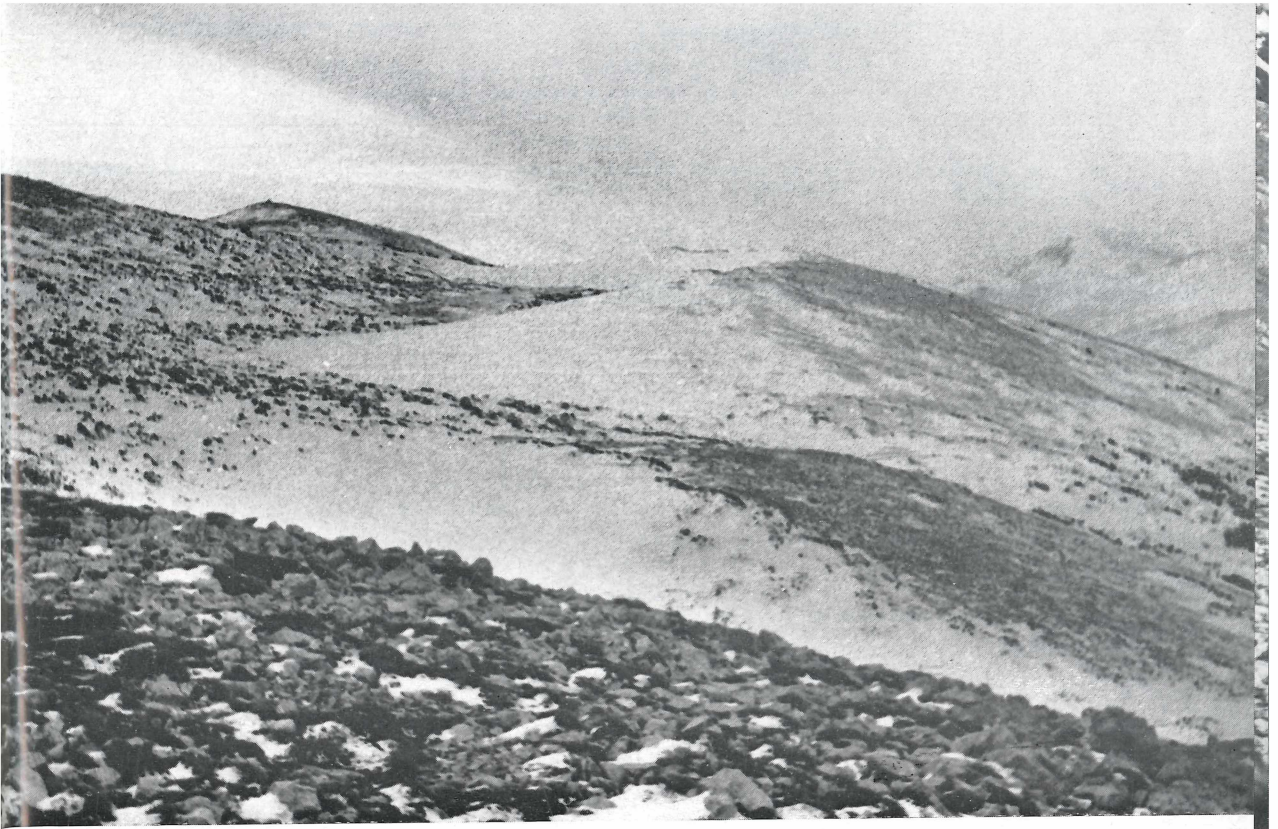
Bild 1: Winteraufnahme, Bild 2: Sommeraufnahme (Raxalpe 1700 m): Deflationsvollformen und Nivationshohlformen
