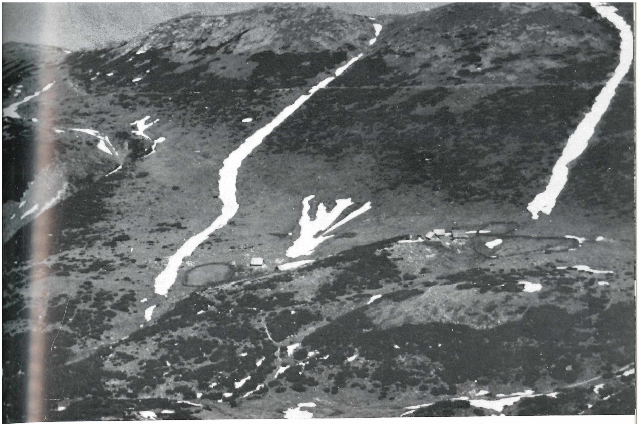
Bild 9: Raxalpe 1700 m bis 1900 m
