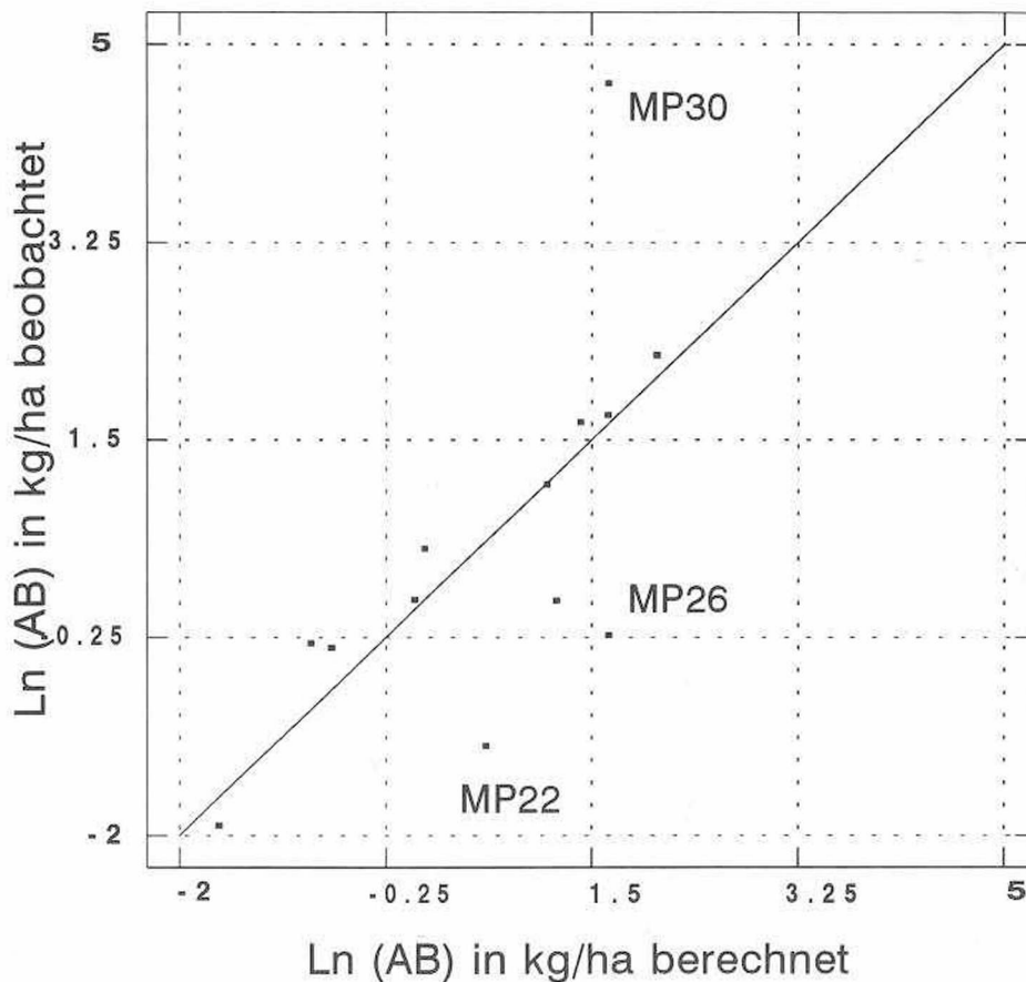
Abb. 3: Streudiagramm der Abtragsregression Brunnen 1991
