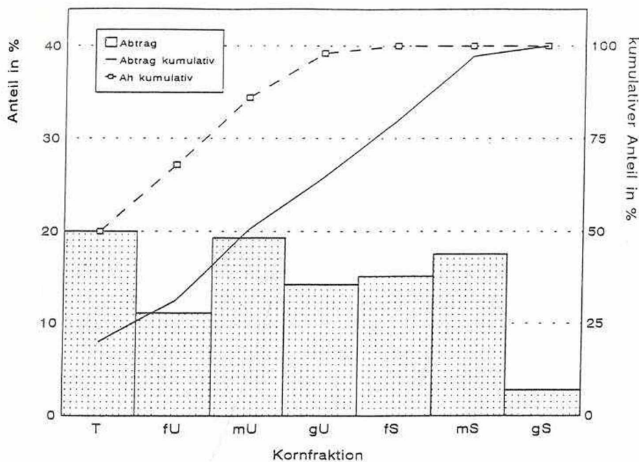
Abb. 5 a: Mittlere Korngrößenverteilung des Abtrags und der Böden in situ auf den Parzellen – a) Grat ; b) Jenner-Süd ; c) Kaser ; d) Brunnen ; e) Weg
