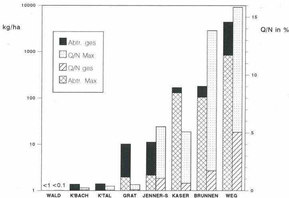
Abb. 1: Abfluß und Abtrag von den Testparzellen 1990 und 1991
