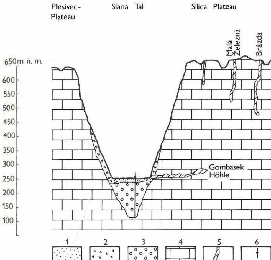
Abb. 3: Schematisches geomorphologisches Profil durch das Tal des Slaná-Flusses 1. Schotter und Sand – Quartär; 2. Fußschuttkegel – Quartär; 3. Schotter und Sand der Poltarformation – Pont; 4. Wettersteinkalke – mittlere Trias; 5. Höhlen; 6. Geologische Bohrungen
