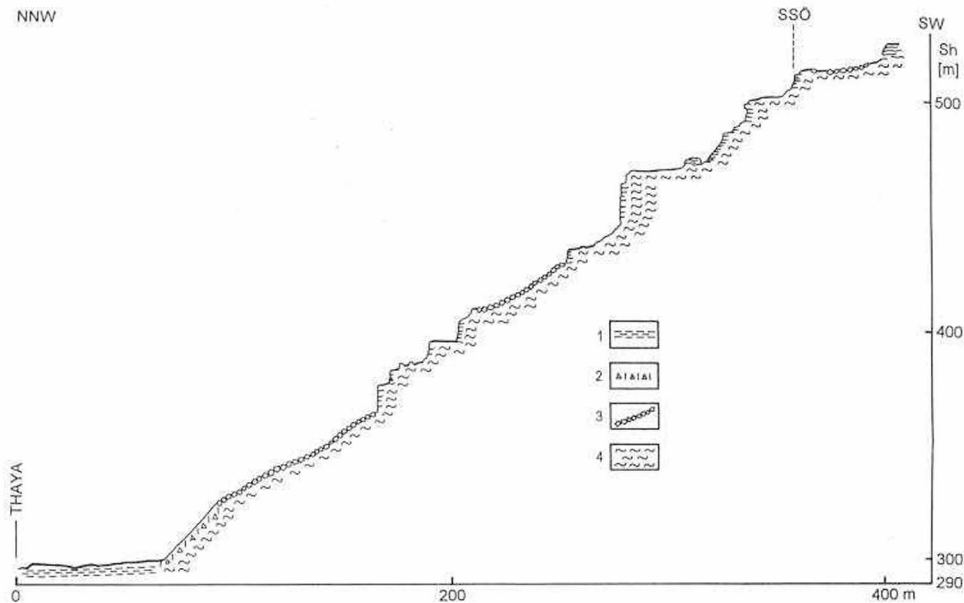
Abb. 2: Querprofil durch den rechten Thayatalhang östlich vom Hügel Býčí hora Erklärungen: 1 – Sedimente der Talaue, 2 – scharfkantiger Hangschutt mit lehmiger Beimischung, 3 – Blockströme, 4 – Orthogneis von Bíteš
