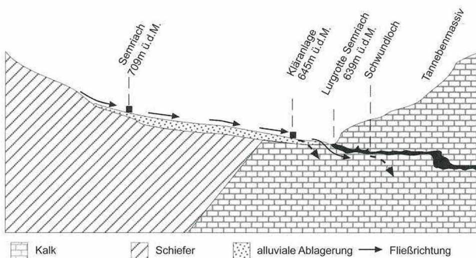
Abb. 4: Schematisches Profil des Border Polje im Raum Semriach
