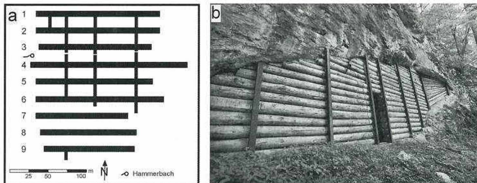
Abb. 6: Karstaspekt Hohlform
