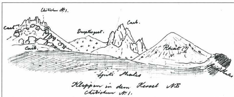
Abb. 3: „Klippen in dem Kessel NE Chitichun Nr. 1“. Geländeskizze aus dem Feldtagebuch von Carl DIENER [fol. 35].
