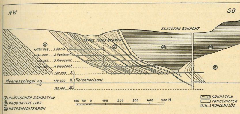
Profil des Franz-Josefs- und St. Stefansschächtes.
