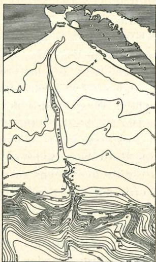
Abb. 5. Karte der submarinen Rinne des Hudson.
