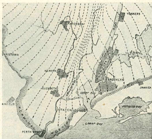
Abb. 2. Die Ausbreitung und Bewegung des Eises zur Zeit der letzten Vergletscherung. Wisconsin-Endmoräne.
