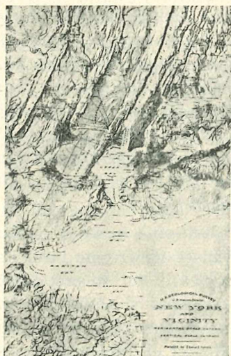
Abb. 7. Relief der Umgebung von Neu-York.
