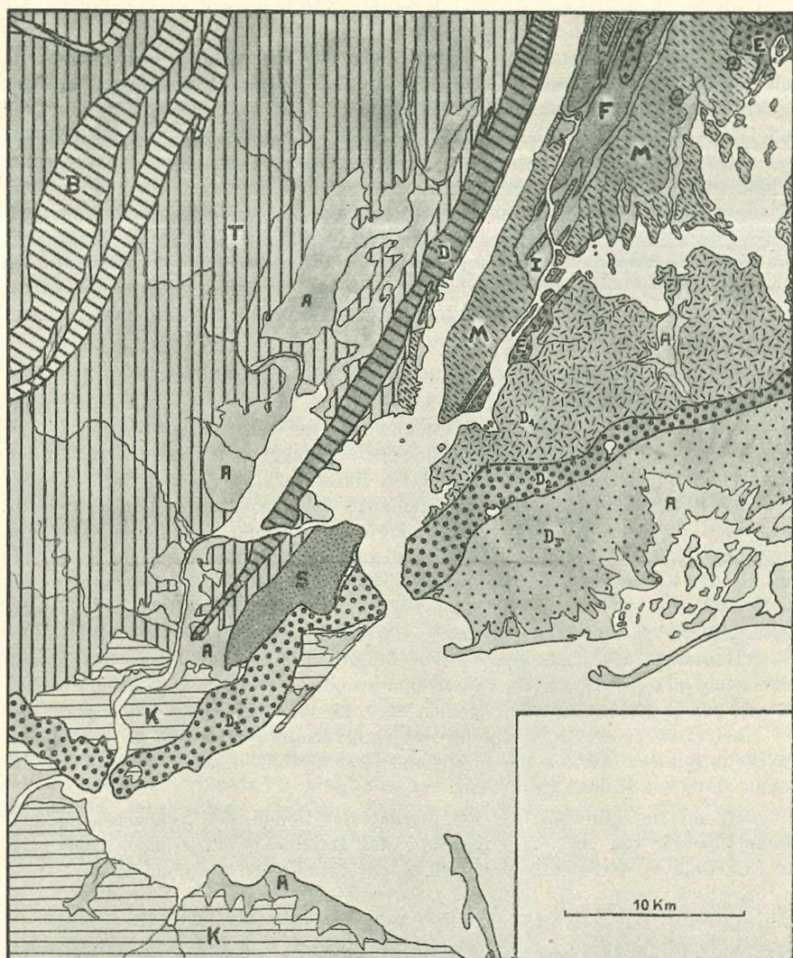
Abb. 1. Geologische Karte der Umgebung von Neu-York.
