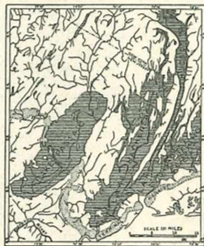
Abb. 4. Rekonstruktion der postglazialen Seen zur Zeit ihrer größten Ausdehnung.
