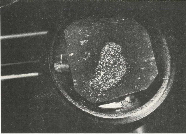
Abb. 2: Gediegen Arsen und Safflorit als „nestförmige“ Imprägnationsvererzung im Rhyodazit von Schweisweiler; Erzanschliff. Vergrößerung: \times 1,5 .
