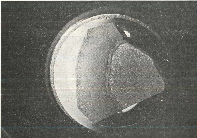
Abb. 4: Carburan und Pechblende (Uraninit) in der Umrandung einer arsenreichen „Erzniere“ im Rhyodazit von Schweisweiler. Vergrößerung: \times 1,5 .
