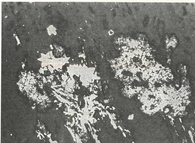
Abb. 9: Safflorit im Erzanschliff als typische Drillings-Kristalle (sogenannte „Safflorit-Sterne“) neben gediegenem Arsen aus dem Rhyodazit von Schweisweiler. Vergrößerung: \times 20 .
