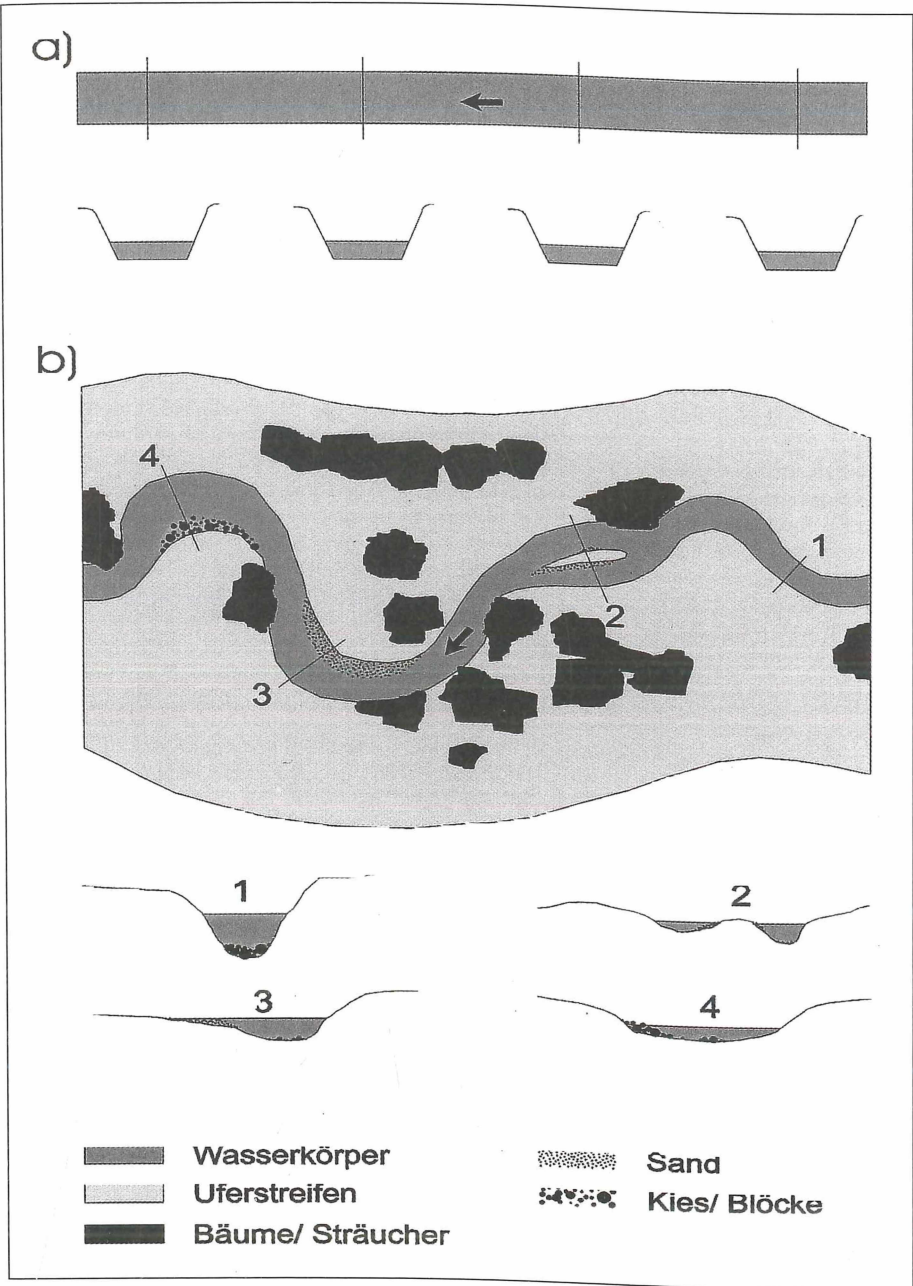
Abb. 9: Vorschlag für die Renaturierung eines Bachabschnittes. (a): begradigter Bach mit Ufer- und Sohlenverbauung. (b): Bach nach erfolgter Renaturierung (verändert nach BLAB 1993)
