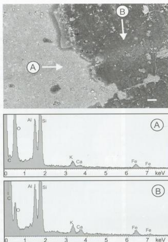
Abbildung 2: Ergebnisse einer semi-quantitativen energie-dispersiven Röntgenquanten-Analyse. Das oberste Bild zeigt eine rückstreuelektronengenerierte Elementkontrastaufnahme (vgl. Abb. 1 I; Maßstab = 20 \mu\text{m} ). Die Positionen an denen die beiden Spektren aufgenommen wurden sind durch Pfeile markiert (A: chemisch schwere Phase; B: chemisch leichte Phase). Besonders auffällig sind die Unterschiede der Kohlenstoff (C) und der Sauerstoff (O) Konzentrationen zwischen den beiden Phasen.
