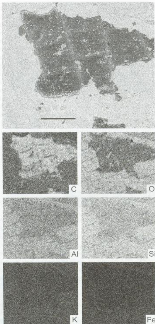
Abbildung 3: Ergebnisse einer Elementkartierung mit Hilfe der energiedispersiven Röntgenquanten-Analyse. Das oberste Bild zeigt eine rückstreuелектронengenerierte Elementkontrastaufnahme (vgl. Abb. 1 F; Maßstab = 200 µm), während die unteren Abbildungen die relativen Häufigkeiten der jeweils angegebenen Elemente auf demselben Objektausschnitt zeigen (je häufiger, desto heller).
