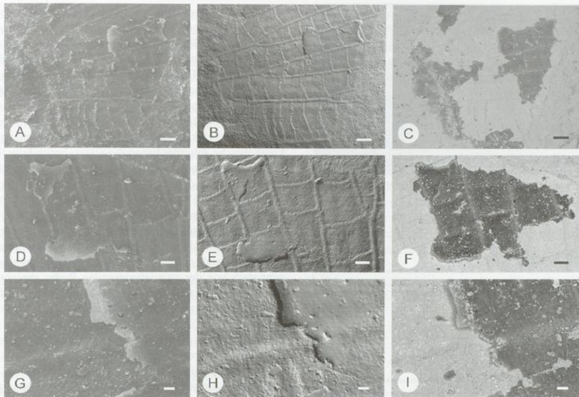
Abbildung 1: Rasterelektronenoptische Aufnahmen eines wahrscheinlich zu den Blatinopsiden gehörenden Flügelfragments von Niedermoschel in verschiedenen Vergrößerungen. A, D, G: Sekundärelektronen Aufnahmen; B, E, H: rückstreuielektronen-generierte Topographiekontrast Aufnahmen; C, F, I: rückstreuielektronen-generierte Element-Kontrast Aufnahmen (A, B, C, Maßstab = 200 \mu\text{m} ; D, E, F, Maßstab = 100 \mu\text{m} ; G, H, I, Maßstab = 20 \mu\text{m} ).
