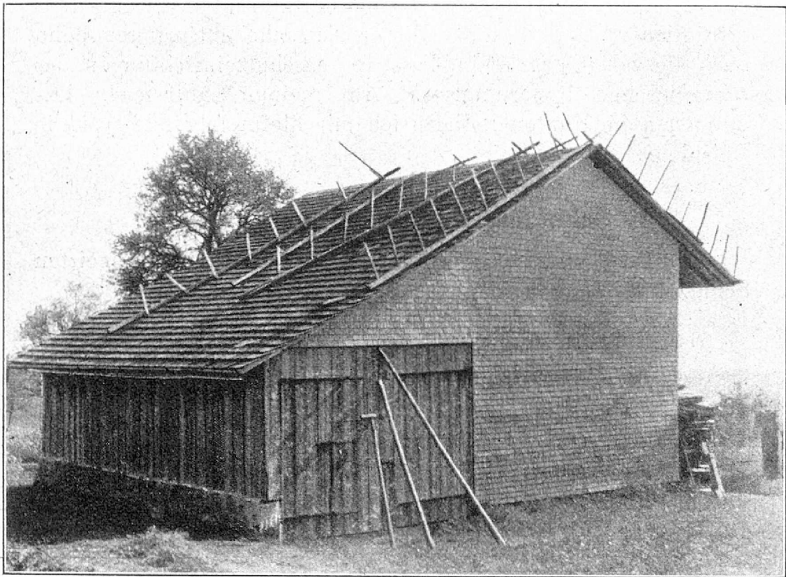
Abb. 2. Haselberg: Windrechen.
