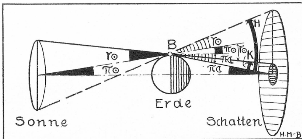
Abb 4 Die Winkel, aus welchen die scheinbaren Radien K des Kerns- und H des Halbschattens berechnet werden.
