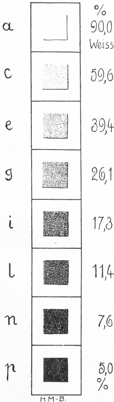
Abb. 10. Grauleiter, d. h. Flächenreihe a—p, deren Helligkeit bezw. Weißgehalt dem Augensehein nach ungefähr gleichmäßig, in Wirklichkeit aber den beigesetzten 0/0-Zahlen nach abnimmt (nach Ostwald).
