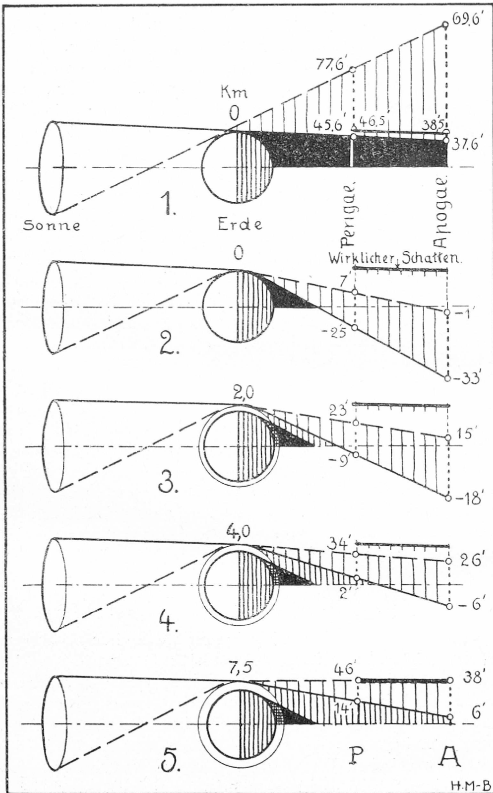
Abb. 11. Die halben Schatten der Erdkugel,
