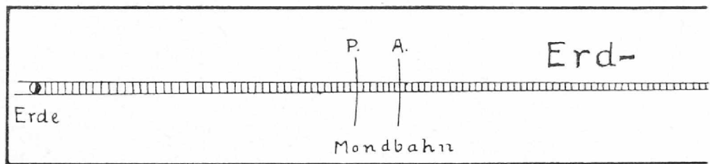
Abb. 12. Erdschatten in wirklichem Verhältnis
