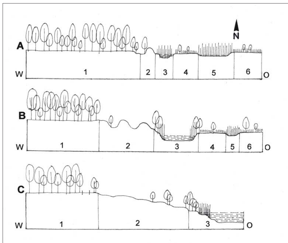
Abb. 6: Geländeprofile (schematisch) entlang einer Kipprippe an verschiedenen Abschnitten durch die Teilflächen 29-48-49 (s. Abb. 2).
