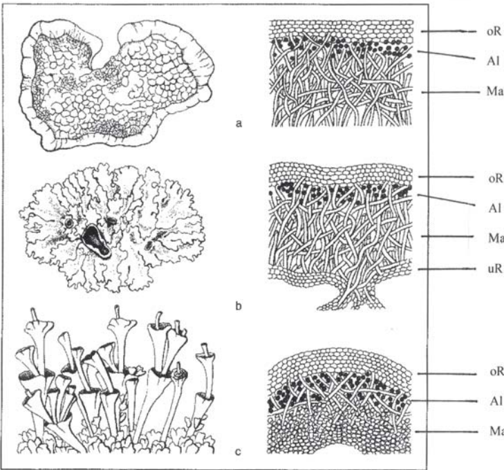
Abb. 50: Wuchsformen und Aufbau von Flechten. a) Krustenflechten, b) Laubflechten, c) Strauchflechten; Al = Algen-schicht, Ma = Mark, oR = obere Rinde, uR = un-tere Rinde (nach SCHÖL-LER 1997).
