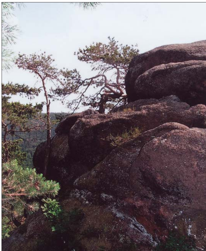
Abb. 7: Granitklippe (Westernklippe). Standort von gesteinsbewohnenden Moosgesellschaften und des Andreaeetum petrophilae .
