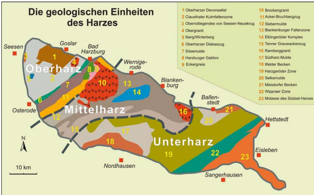
Abb. 3: Geologische Übersichtskarte des Harzes (RAPSILBER et al. 2006).
