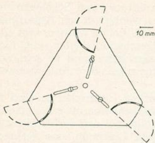
Abb. 2. Schalen-Windmesser, Aluminiumplatte des Schalensystems. Schalen aus halben Tischtennisbällen gestrichelt.
