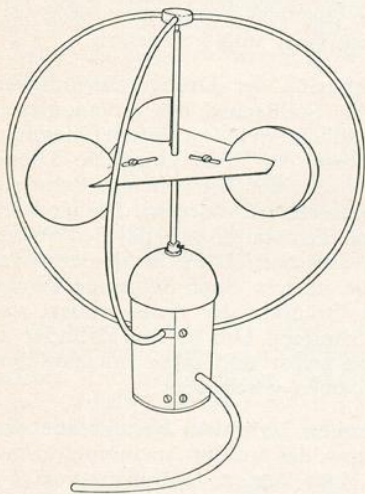
Abb. 1. Schalen-Windmesser, Fühlgerät.
