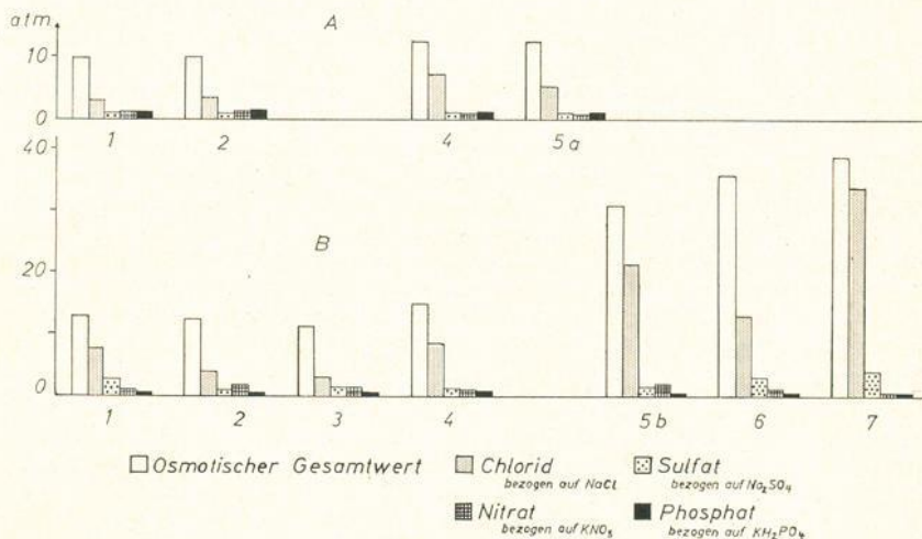
Abb. 1. Preßsaftanalysen von Blättern einiger Spülsaum-, Primär- und Sekundärdünenpflanzen. A = Langeoog; B = Vari. 1 = Cakile maritima , 2 = Salsola kali , 3 = Polygonum maritimum , 4 = Agropyron junceum , 5a = Elymus arenarius , 5b = Diotis maritima , 6 = Atriplex tatarica , 7 = Salicornia herbacea (als Vergleich toniger Salzböden)
