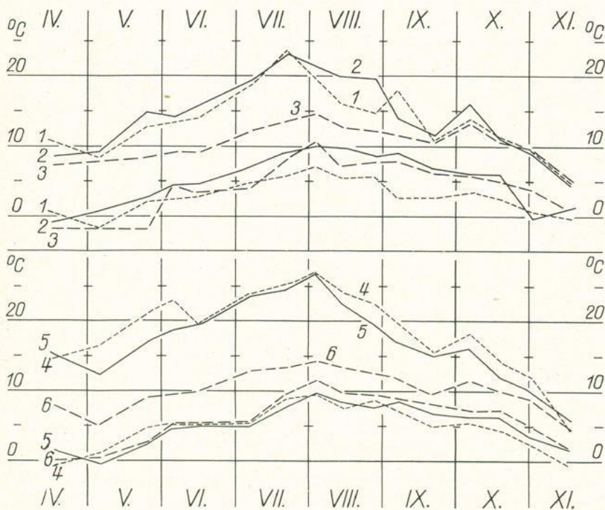
Abb. 2. Extremtemperaturen von April bis November 1967 in 1 bis 2 cm Bodentiefe
