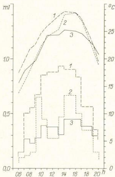
Abb. 3. Evaporation und Lufttemperatur in 20 bis 30 cm Höhe an einem sehr warmen, sonnigen Sommertag (19.7.67) über Sphagnetum medii (1) und Piceo-Vaccinietum uliginosi (2) im Vergleich zum benachbarten Calamagrostio villosae-Piceetum (3).
