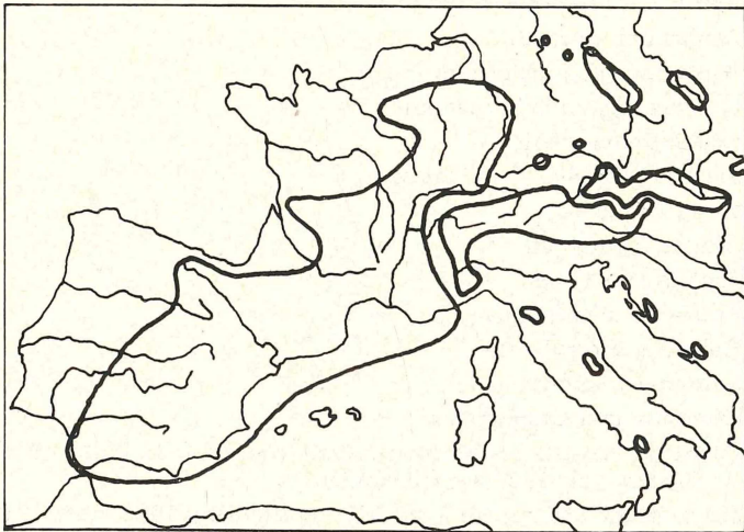
Abb. 1. Verbreitung von Biscutella Subsektion Laevigatae (nach HEGI)
