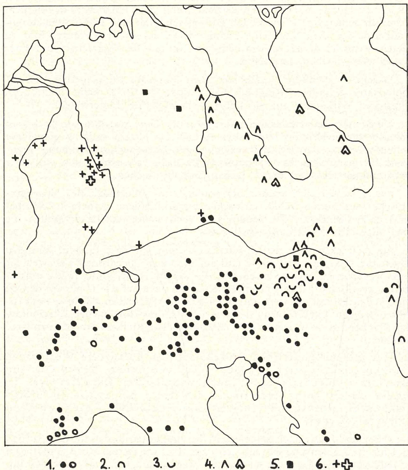
Abb. 2. Die Gliederung des Verbreitungsgebietes des Brillenschötlchens ( Biscutella laevigata L.) in Mitteleuropa, nach MACHATSCHKI-LAURICH (1926) und MANTON (1934 und 1937). Ausgefüllte Zeichen bedeuten durch zytologische Untersuchung sicher als diploid bzw. tetraploid erkannte Formen, nicht ausgefüllte Zeichen Formen, für welche Diploide bzw. Tetraploide noch nicht nachgewiesen, sondern nur zu vermuten sind. 1. Tetraploide Formen. — 2.— 6. Diploide Formen: 2. Unterart austriaca ; 3. Var. mollis der Unterart austriaca ; 4. Formenreihe der Unterarten kernerii und gracilis ; 5. Unterarten guestphalica (Hohenstein) und tenuifolia (Nordhausen); 6. Formenreihe der Unterart alsatica . (Aus EBERLE 1949.)
